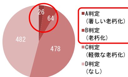
<県管理31漁港における漁港施設の老朽化進行状況（H29末）>
