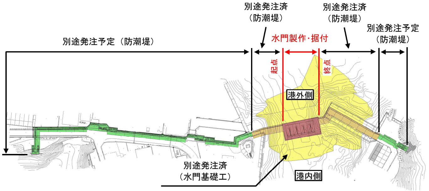
計画平面図
