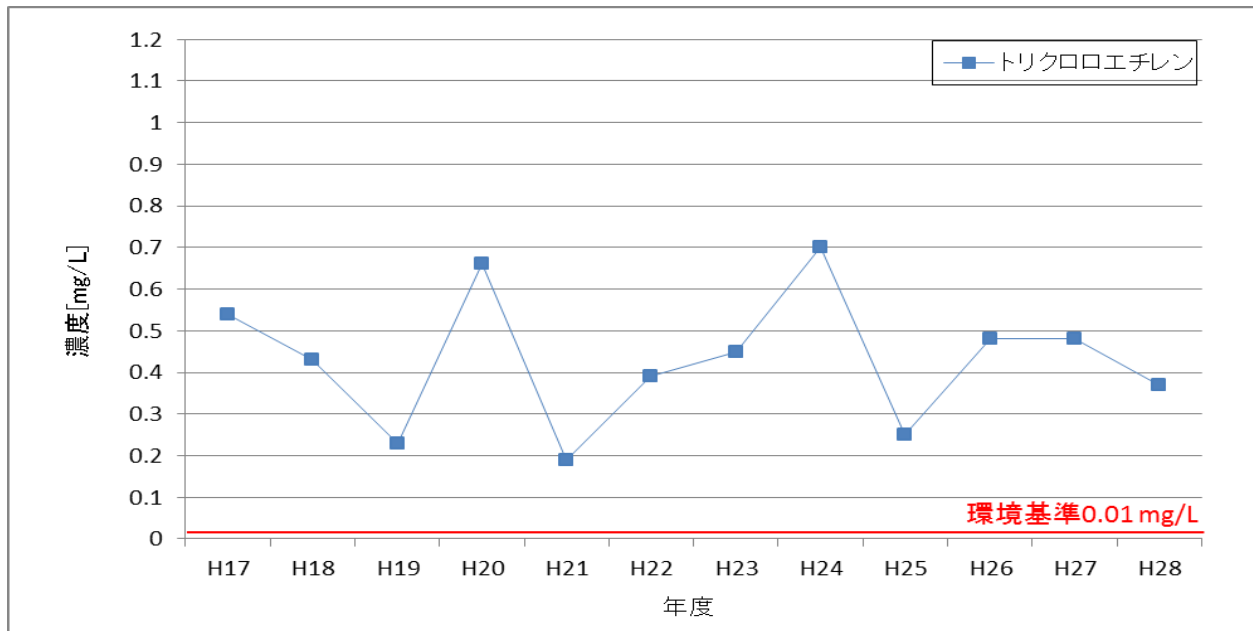
図2-2-1: 花巻市北寺林(2052010000100)におけるトリクロロエチレン濃度の経年変化
