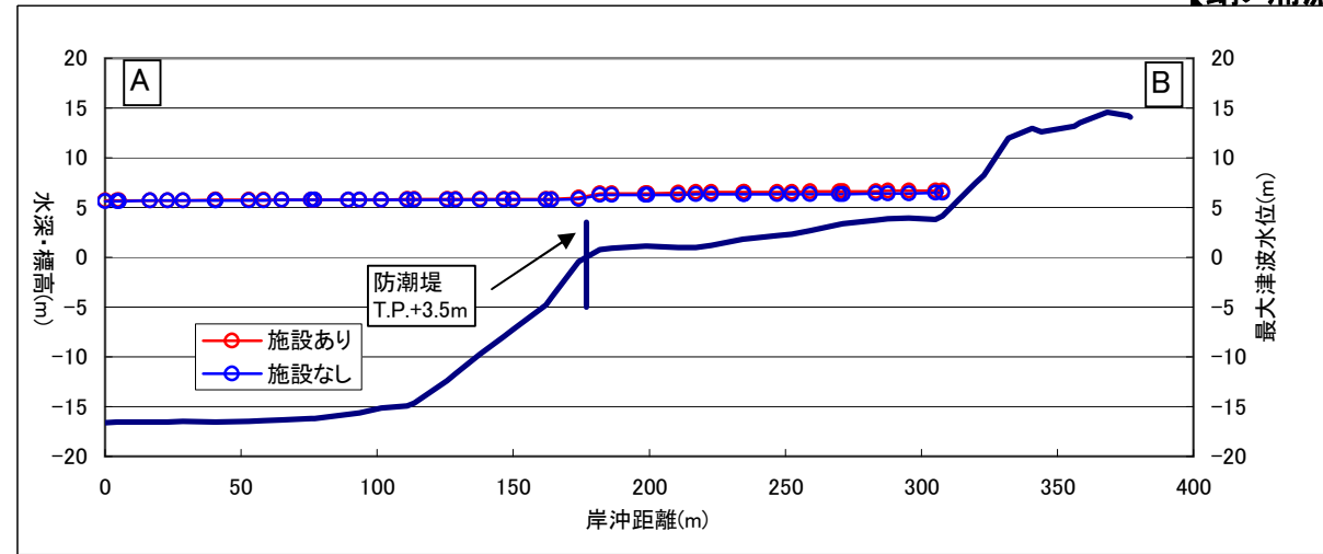
図3.5 津波最大水位
