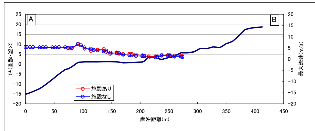
図3.36 津波最大流速
