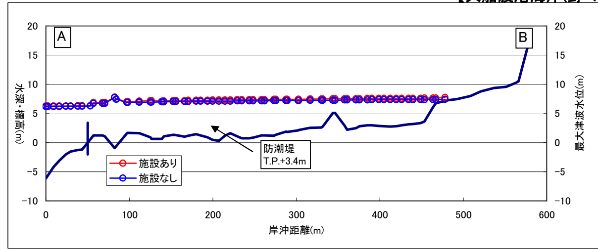
図3.30 津波最大水位
