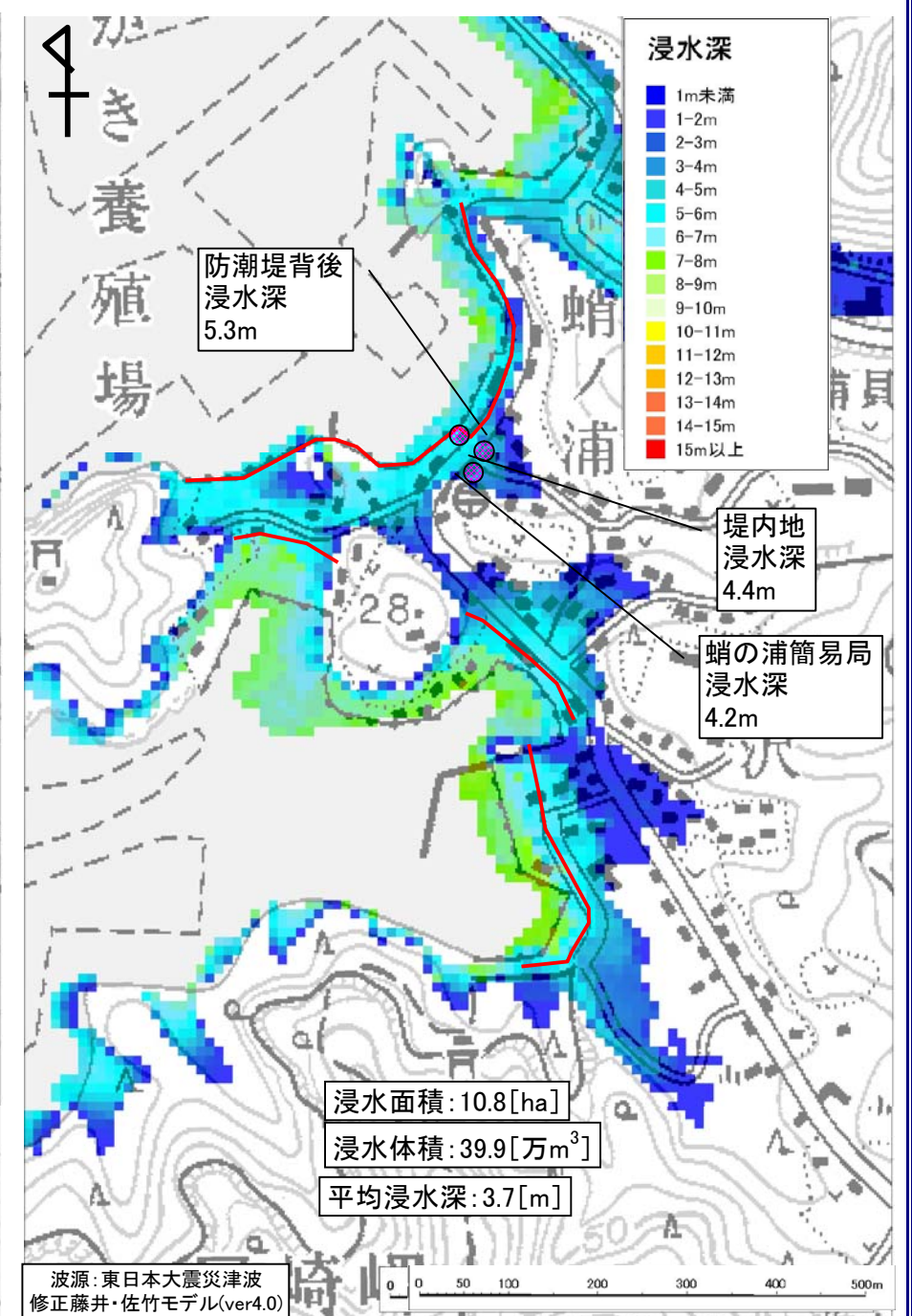
図6.5 浸水深平面分布図
