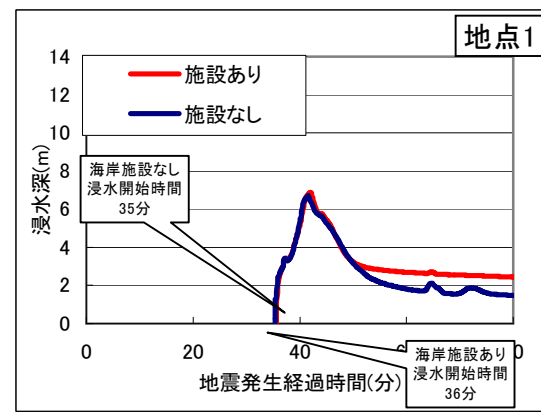
図3.32(1) 評価ポイント(防潮堤背後)における浸水深時系列分布図
