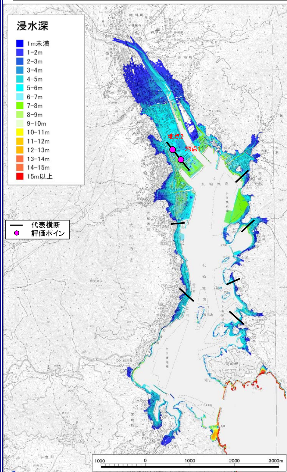
図3.1 浸水深平面分布図(施設なし)
