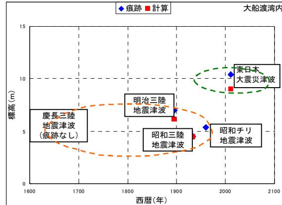
図4.2 既往津波別、地区毎の最大津波水位
