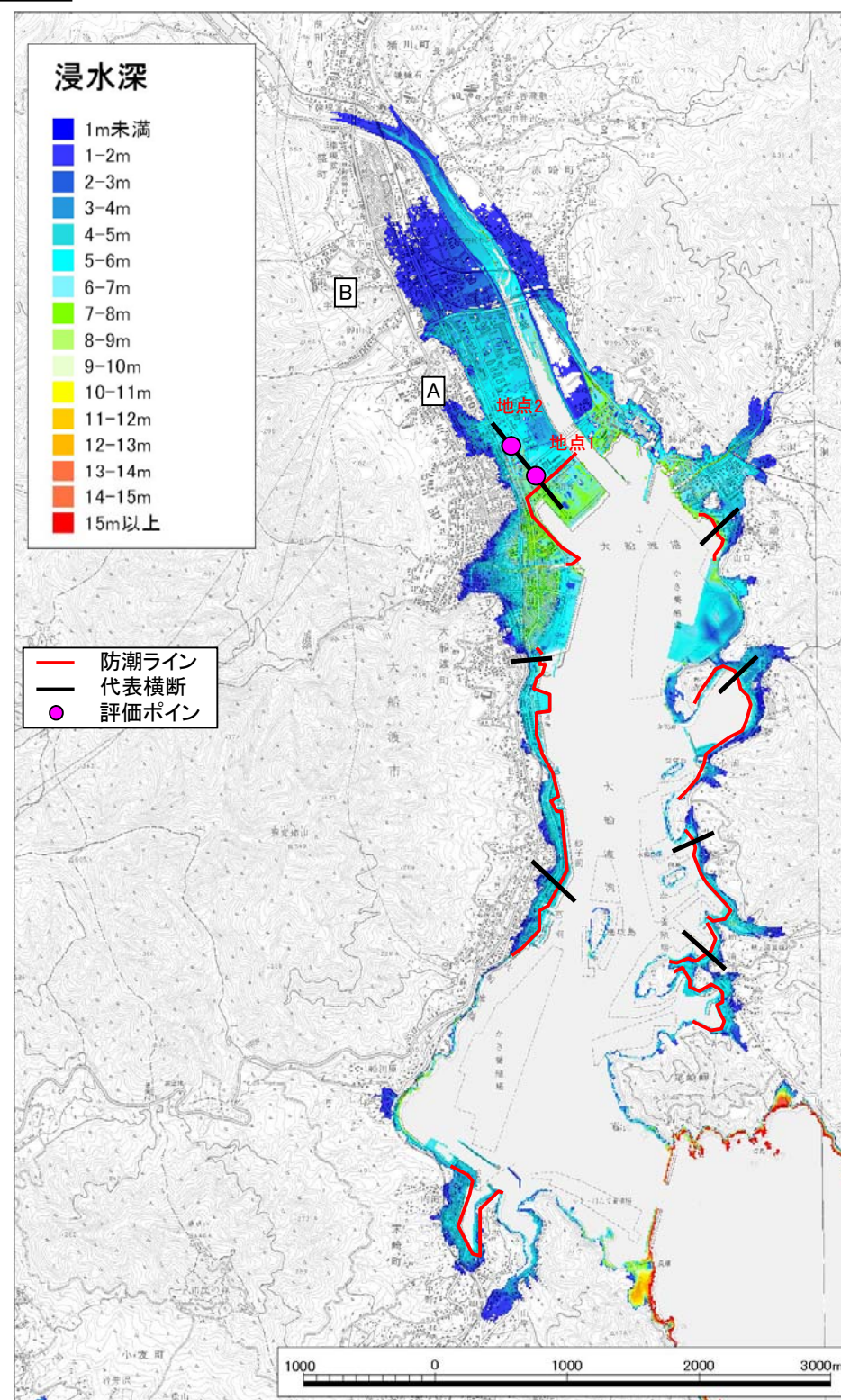
図3.2 浸水深平面分布図(施設あり)
