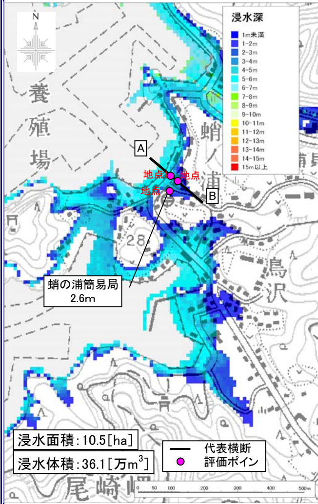
図3.3 浸水深平面分布図(施設なし)
