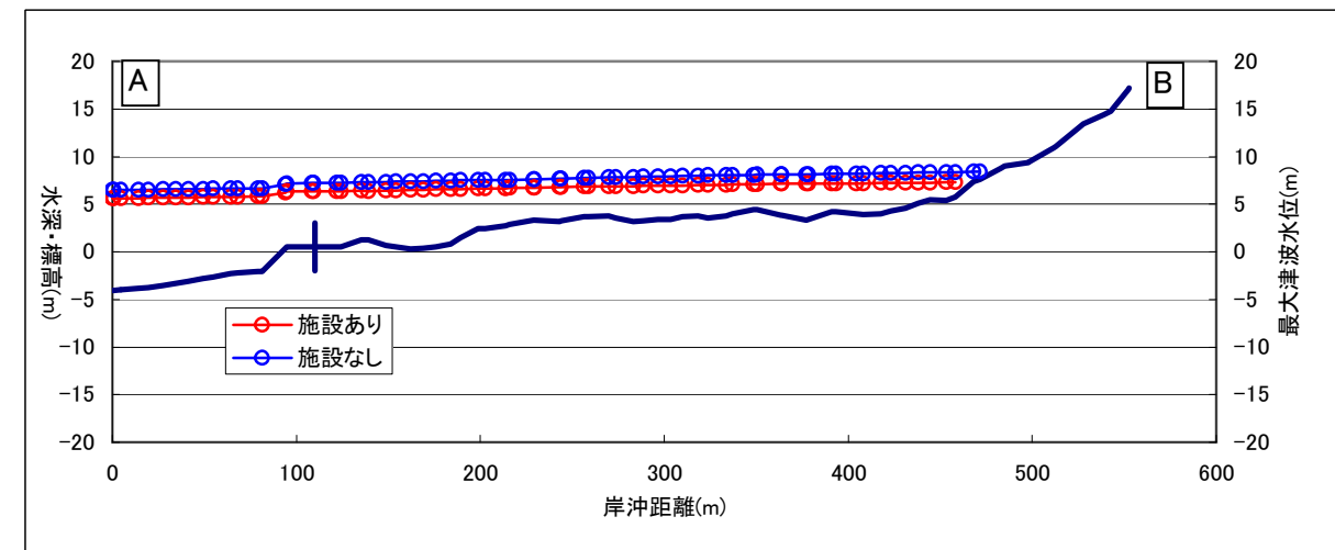
図3.16 津波最大流速
