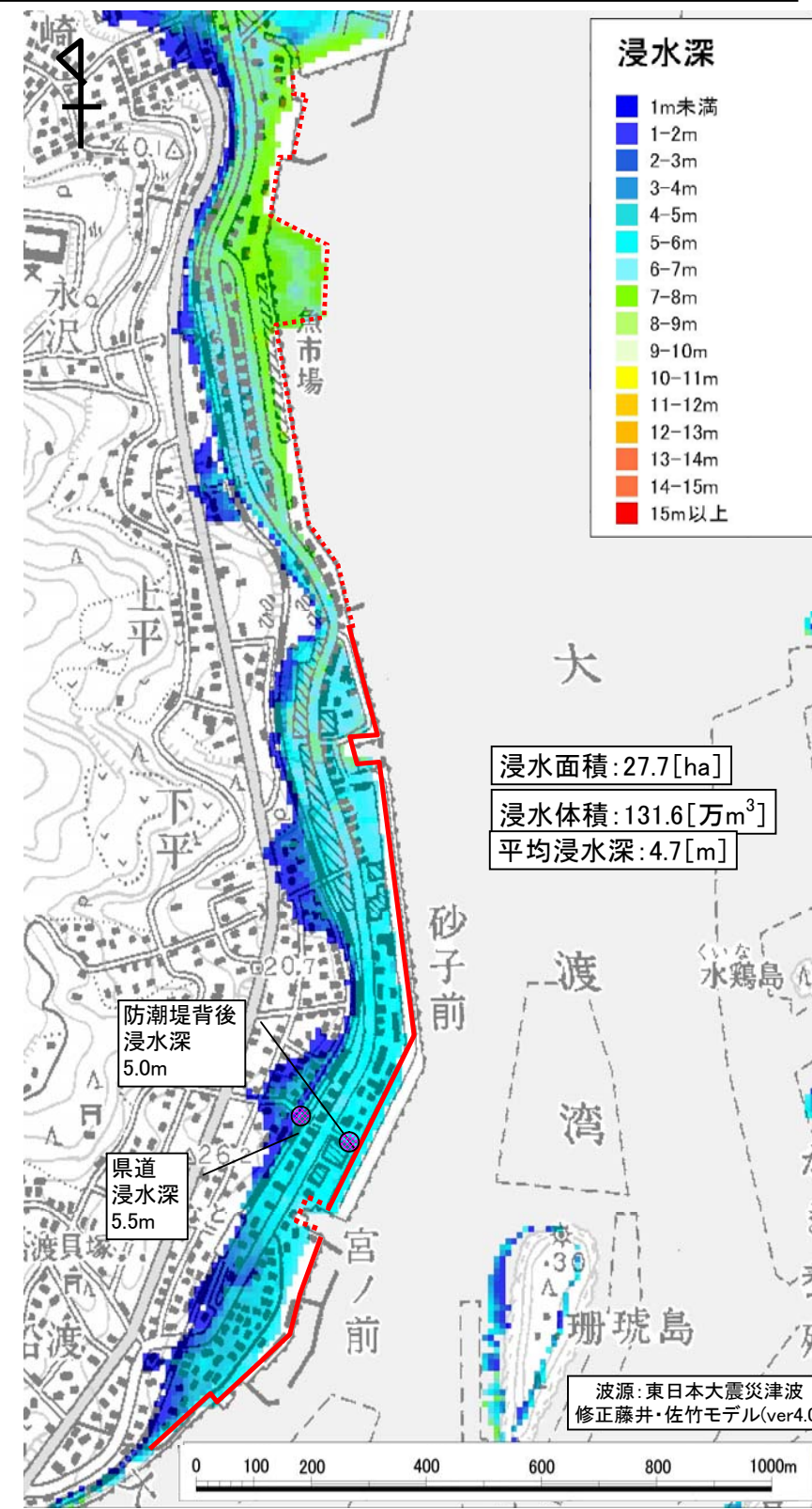
図6.14 浸水深平面分布図
