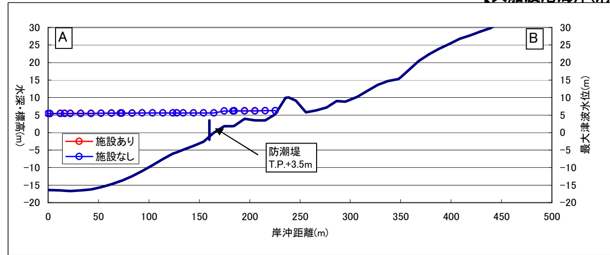
図3.10 津波最大水位
