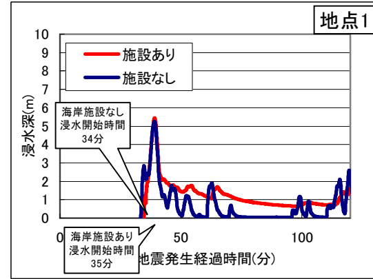
図3.7(1) 評価ポイント(防潮堤背後)における浸水深時系列分布図
