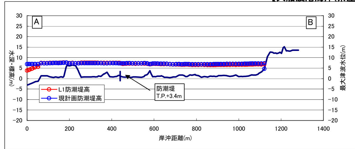
図3.25 津波最大水位
