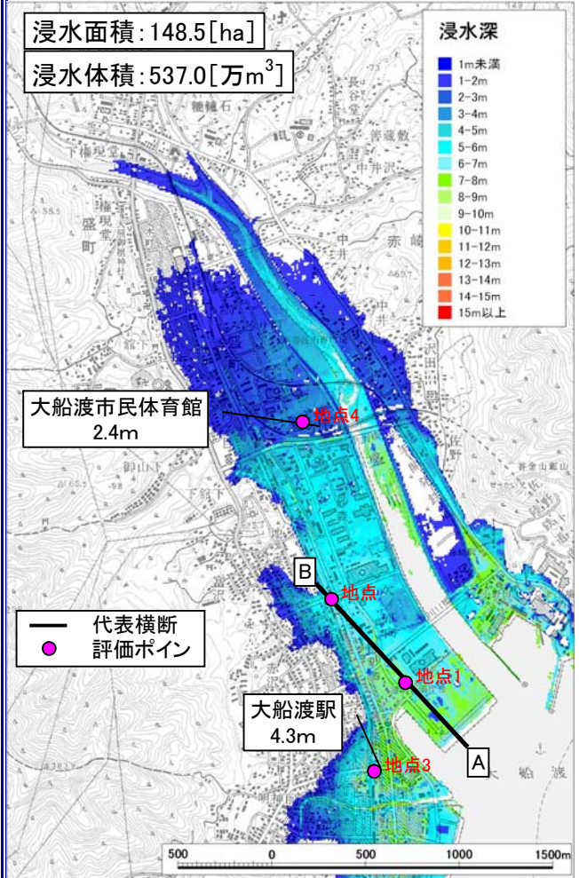
図3.23 浸水深平面分布図(施設なし)
