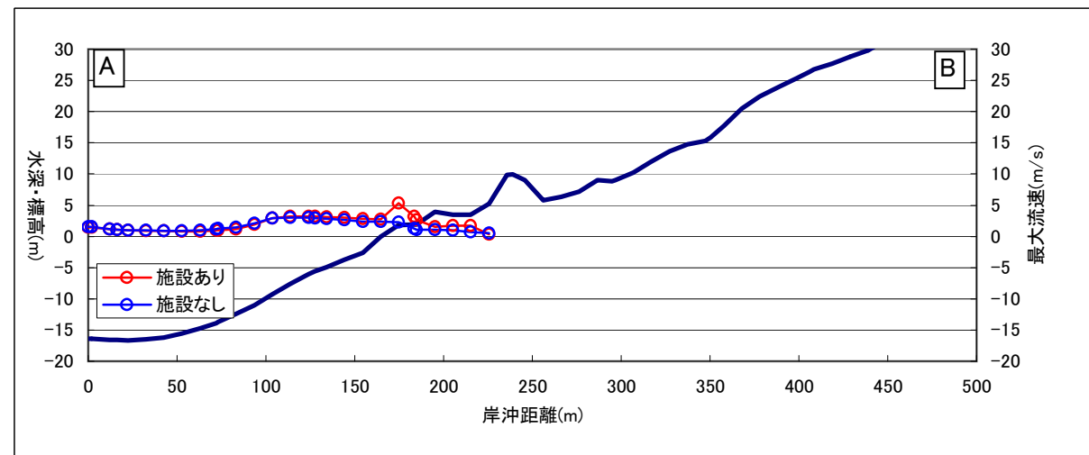
図3.11 津波最大流速
