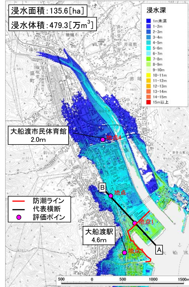
図3.24 浸水深平面分布図(施設あり)
