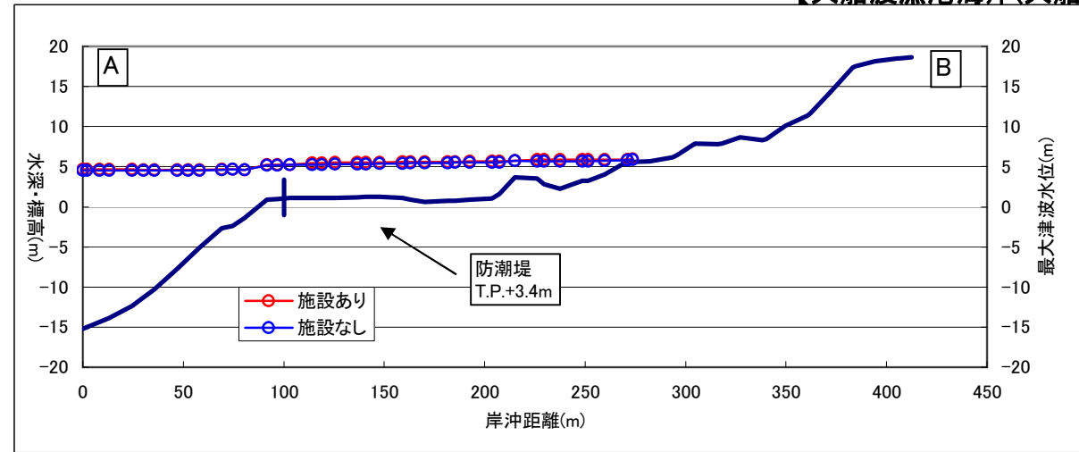
図3.35 津波最大水位
