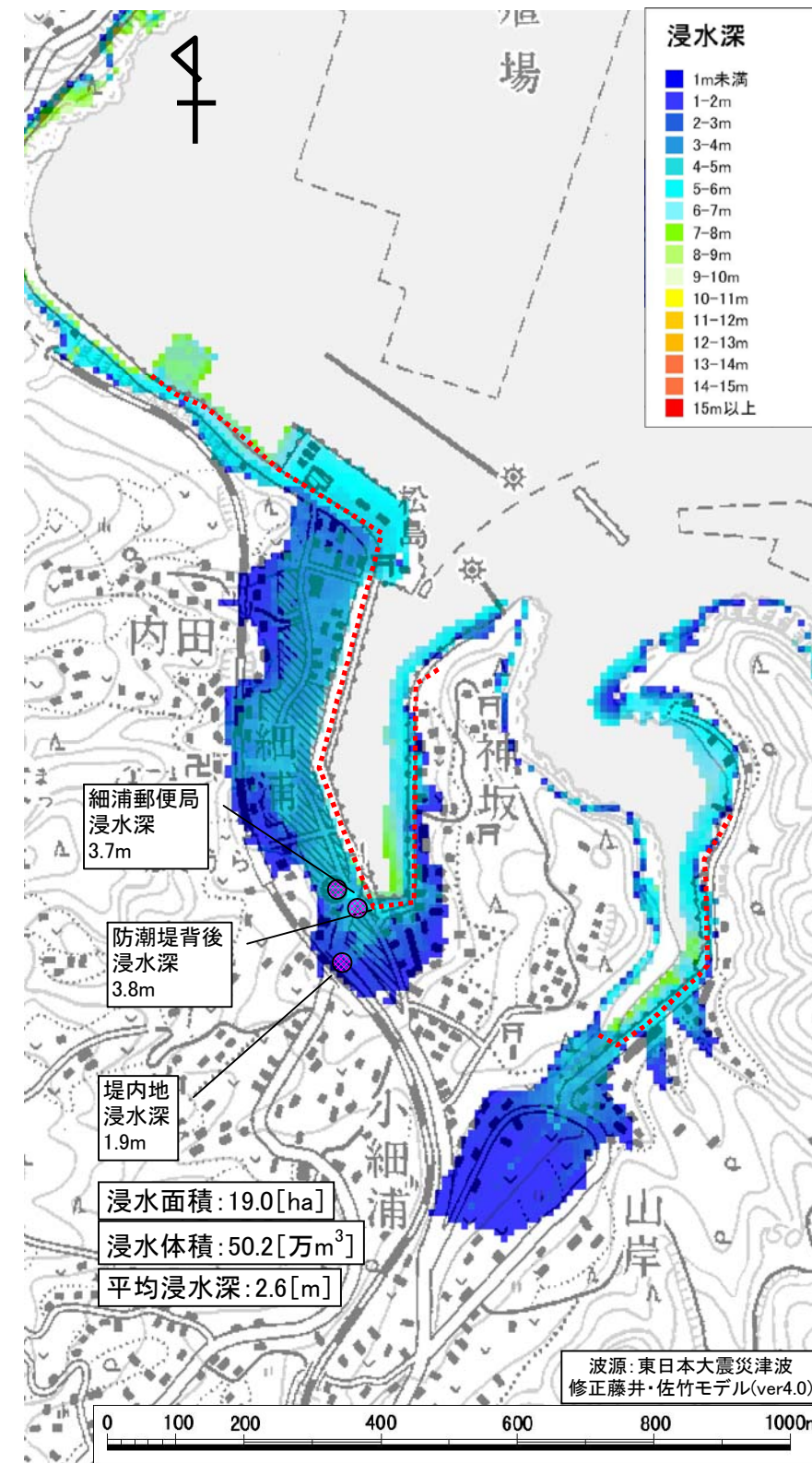
図6.17 浸水深平面分布図
