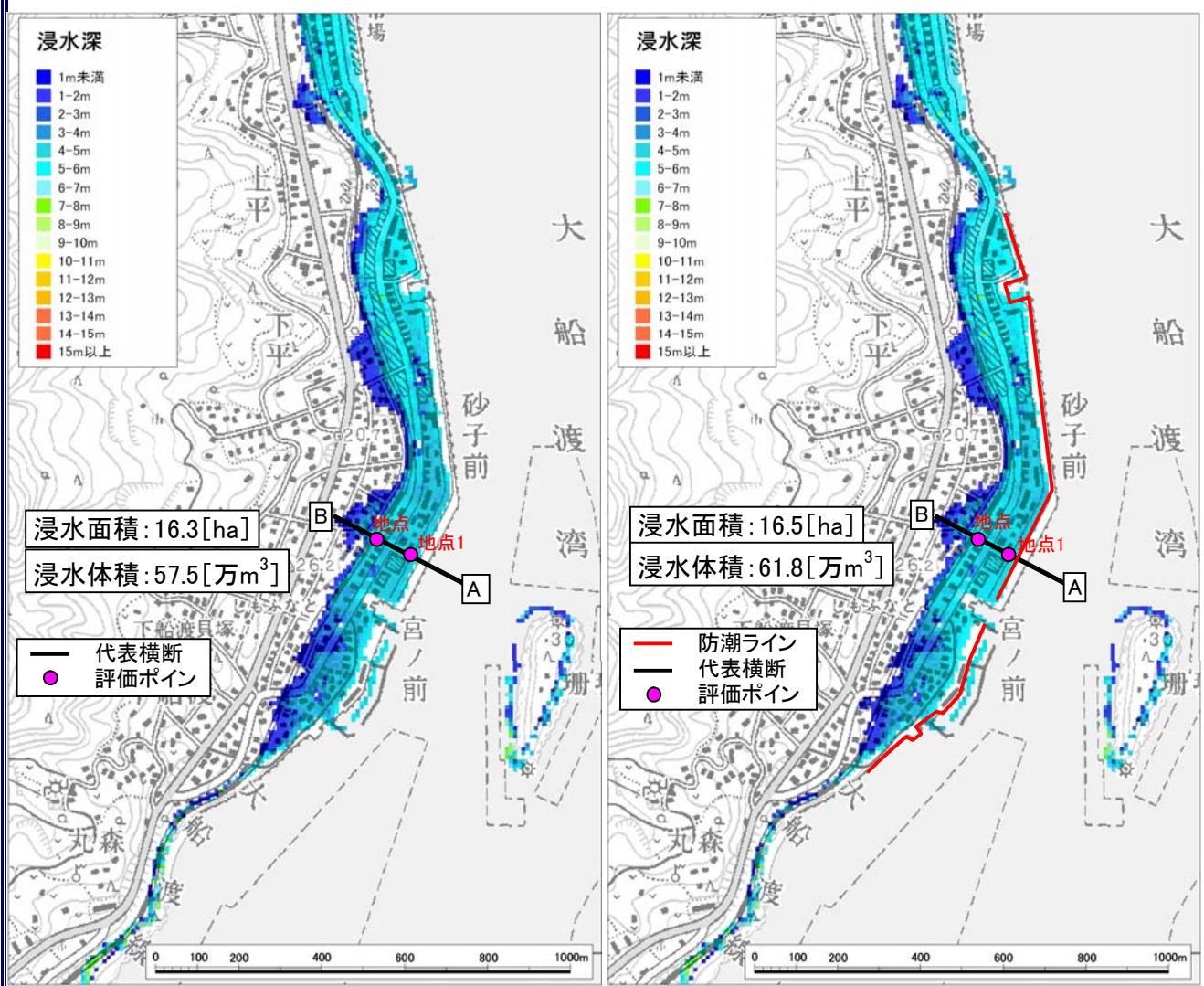
図3.33 浸水深平面分布図(施設なし)
