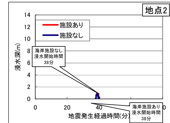
図3.12(2) 評価ポイント(堤内地)における浸水深時系列分布図
