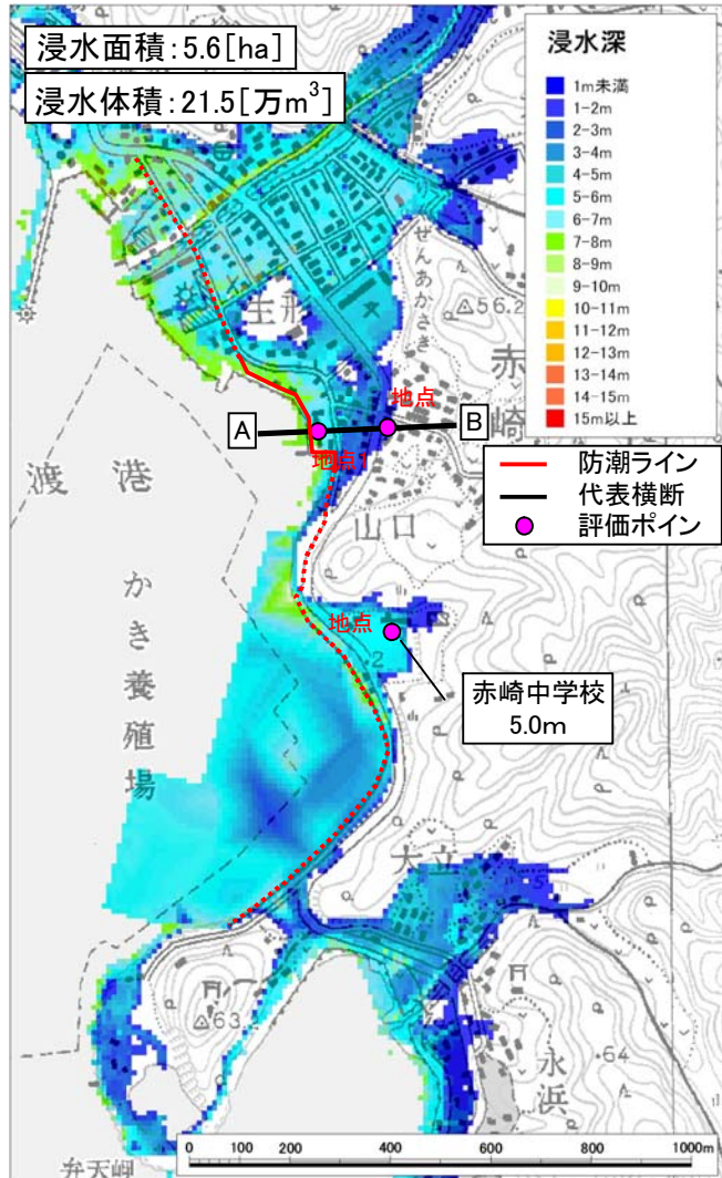
図3.19 浸水深平面分布図(施設あり)
