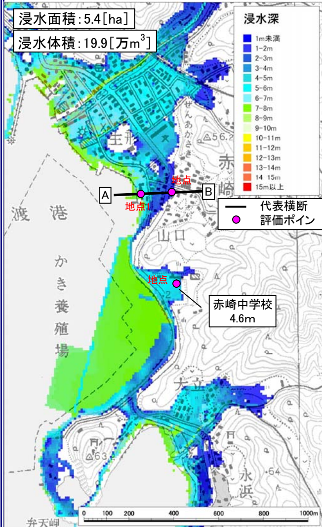
図3.18 浸水深平面分布図(施設なし)
