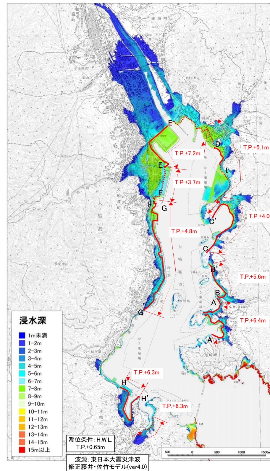
図6.2 浸水深平面分布図
