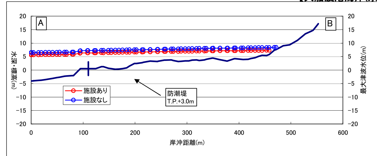
図3.15 津波最大水位
