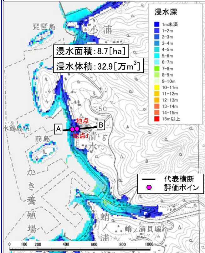
図3.8 浸水深平面分布図(施設なし)
