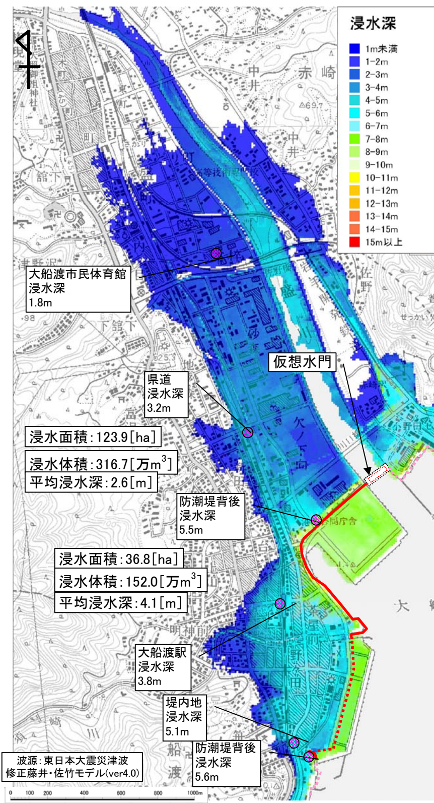
図6.10 浸水深平面分布図
