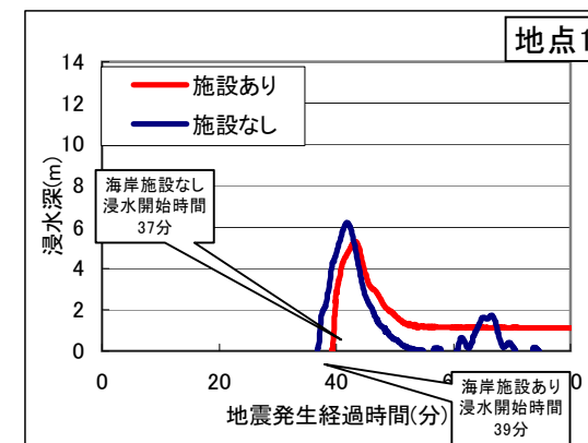
図3.17(1) 評価ポイント(防潮堤背後)における浸水深時系列分布図
