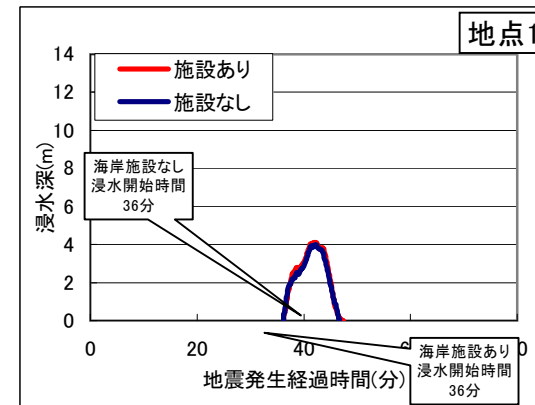
図3.22(1) 評価ポイント(防潮堤背後)における浸水深時系列分布図
