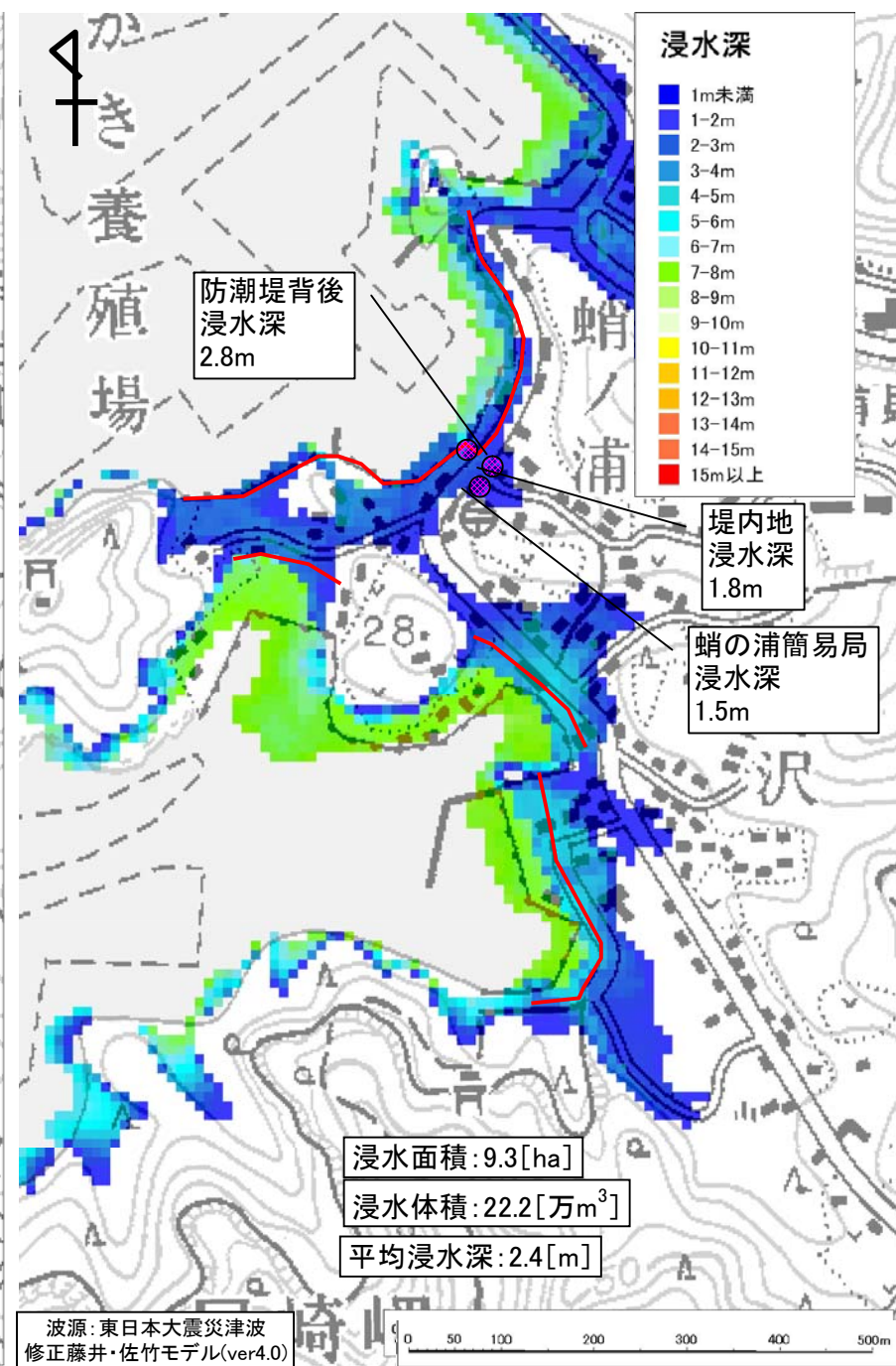
図6.4 浸水深平面分布図
