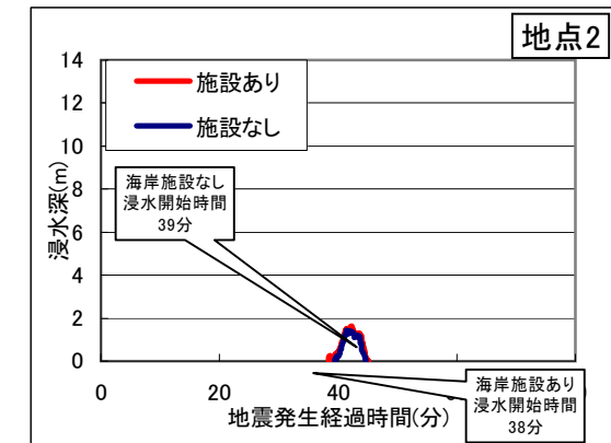
図3.22(2) 評価ポイント(堤内地)における浸水深時系列分布図
