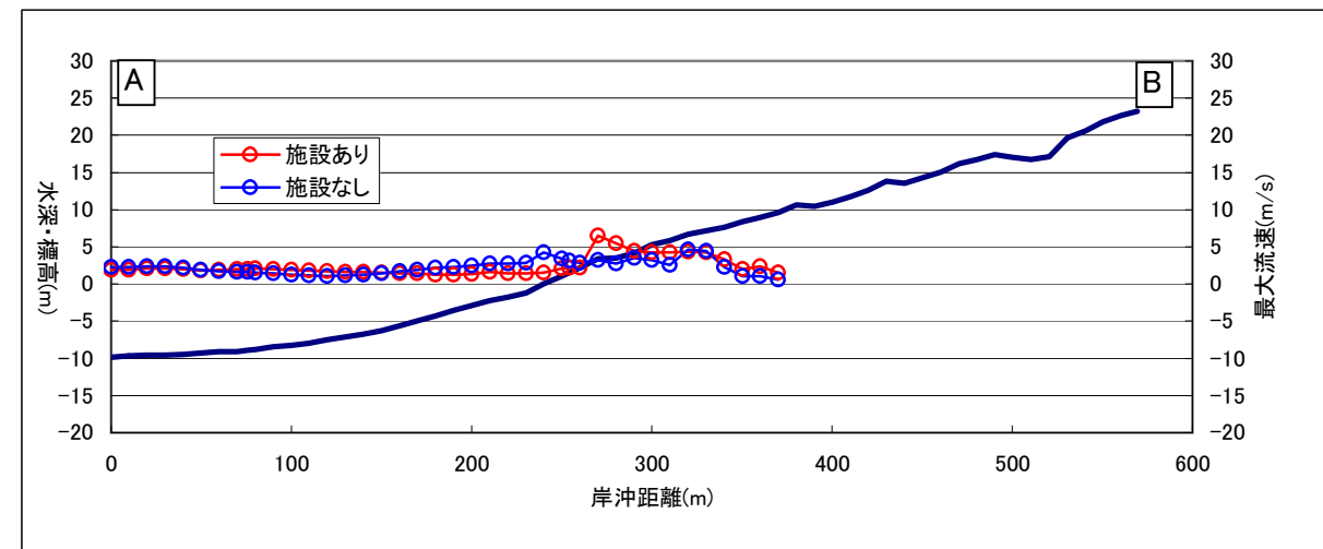
図3.21 津波最大流速
