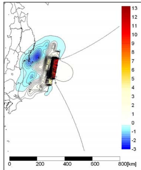
図2.2 初期地盤変動量
