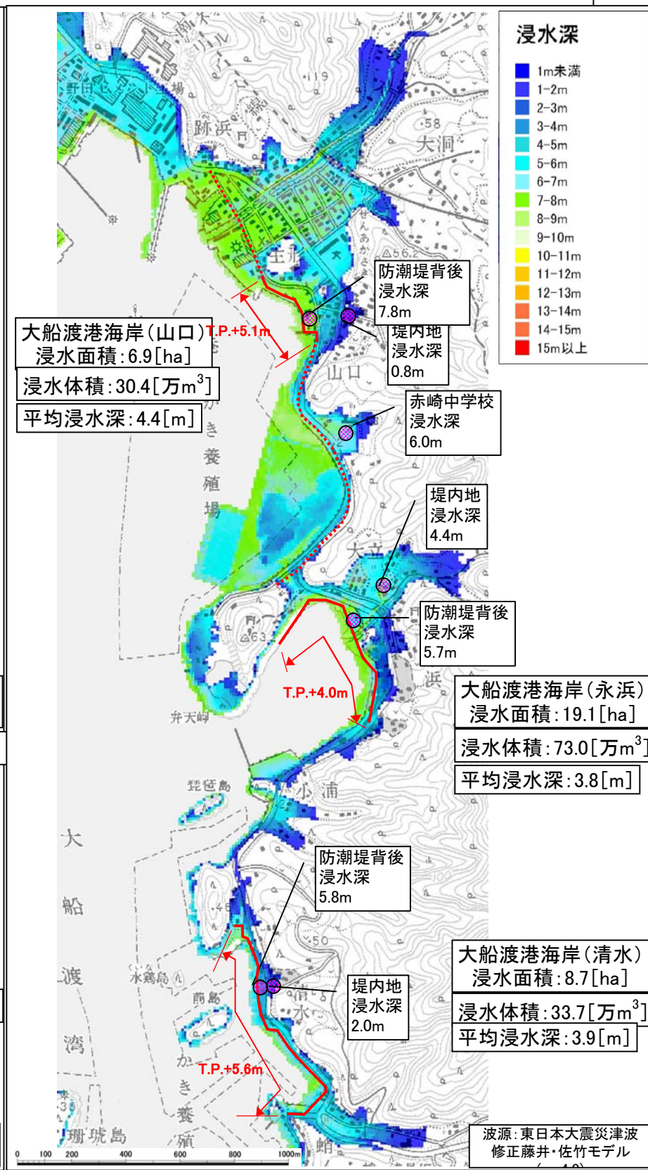
図6.8 浸水深平面分布図
