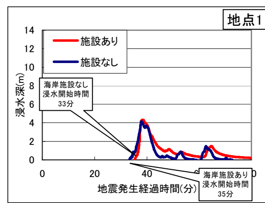
図3.37(1) 評価ポイント(防潮堤背後)における浸水深時系列分布図
