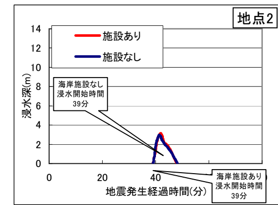
図3.32(2) 評価ポイント(堤内地)における浸水深時系列分布図
