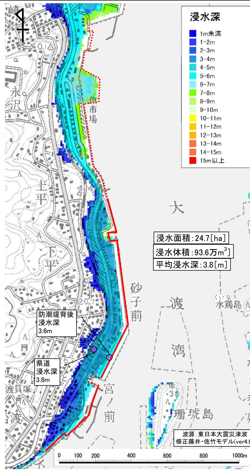
図6.13 浸水深平面分布図
