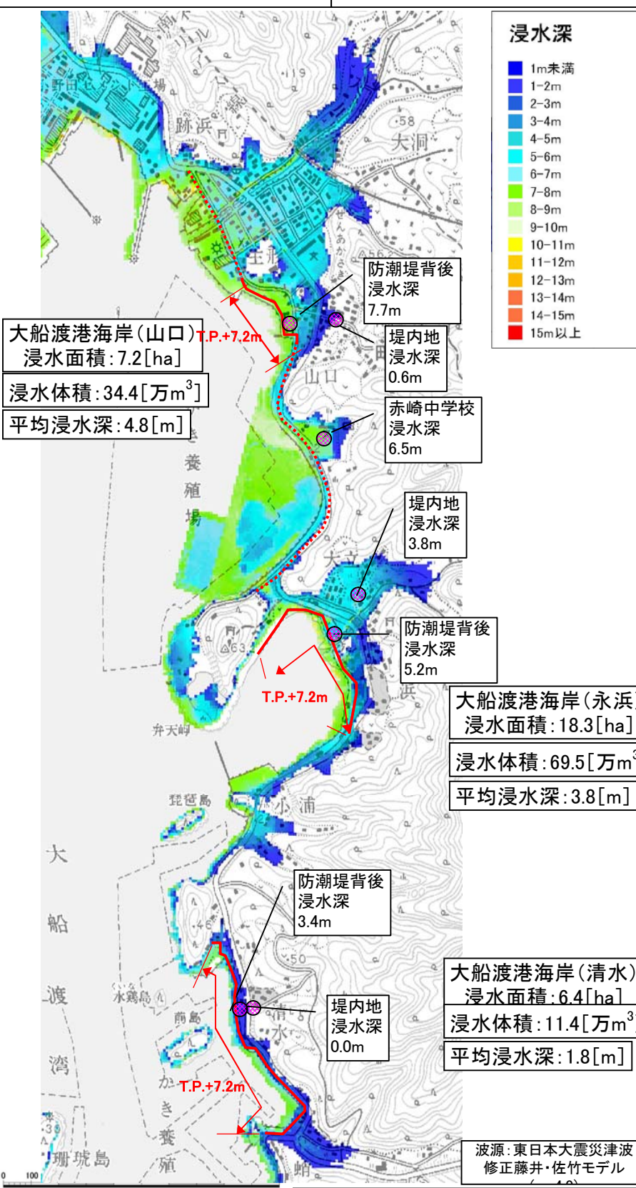
図6.7 浸水深平面分布図
