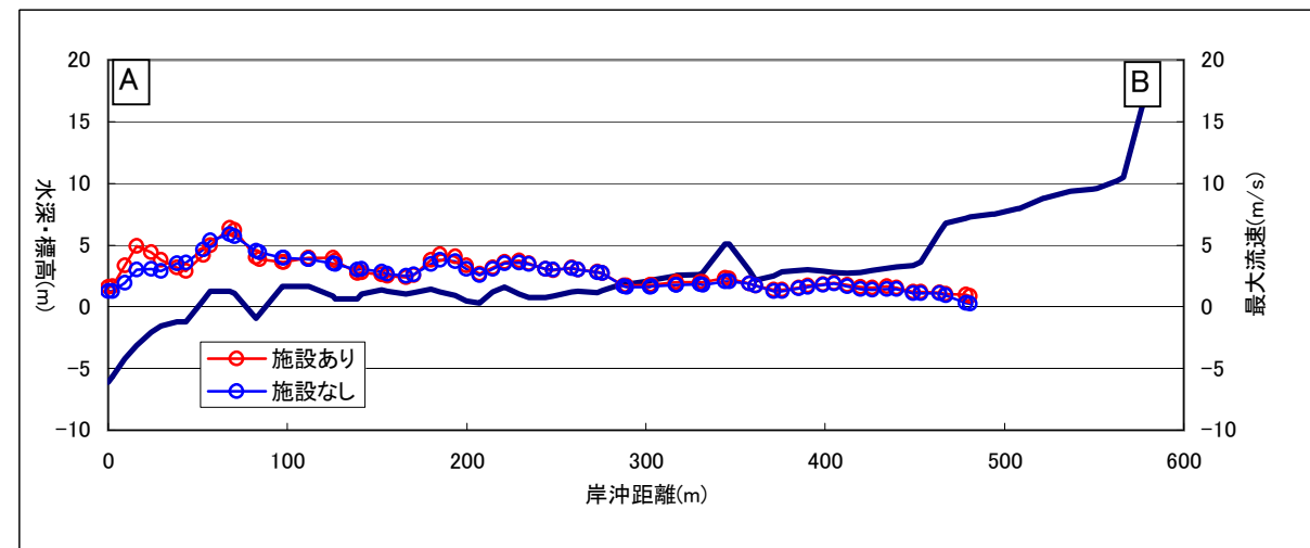
図3.31 津波最大流速
