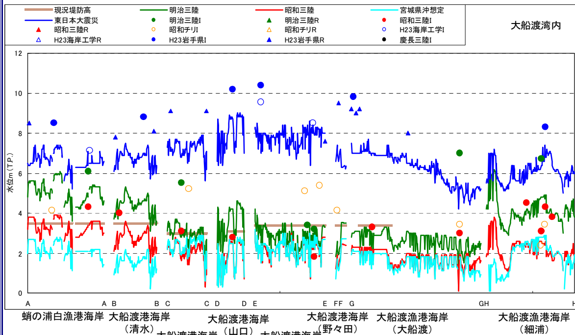
図4.2 既往津波別、地区毎の最大津波水位
