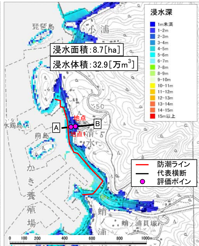
図3.9 浸水深平面分布図(施設あり)
