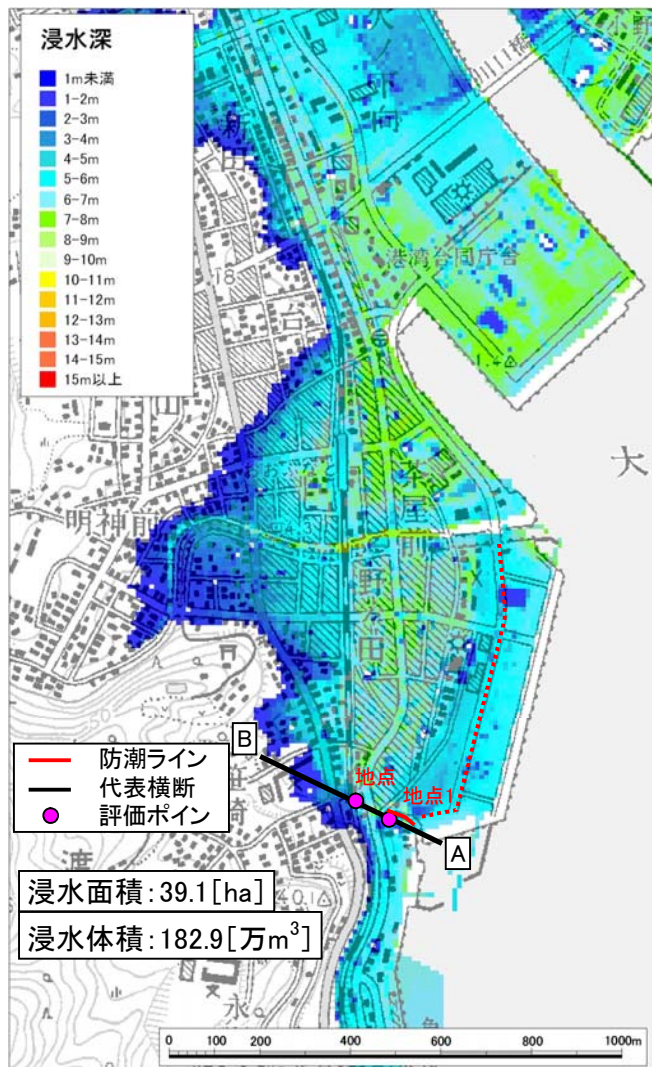
図3.29 浸水深平面分布図(施設あり)
