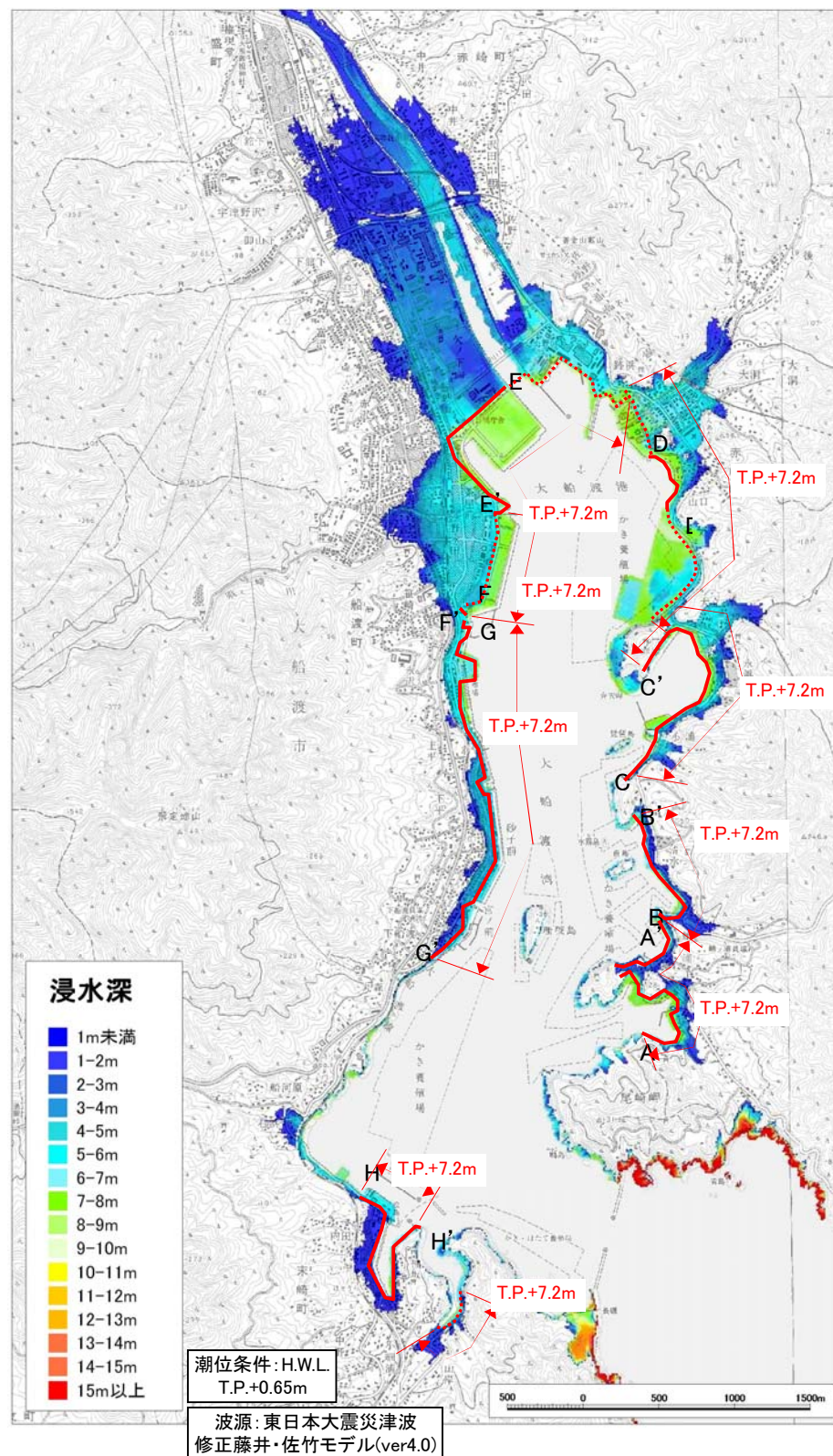
図6.1 浸水深平面分布図
