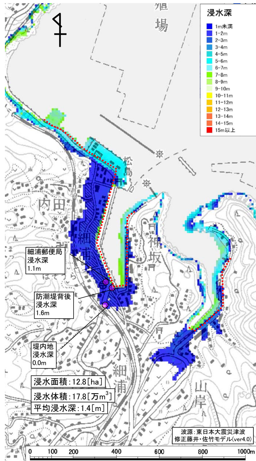
図6.16 浸水深平面分布図
