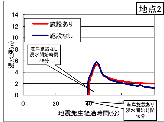
図3.27(2) 評価ポイント(堤内地)における浸水深時系列分布図
