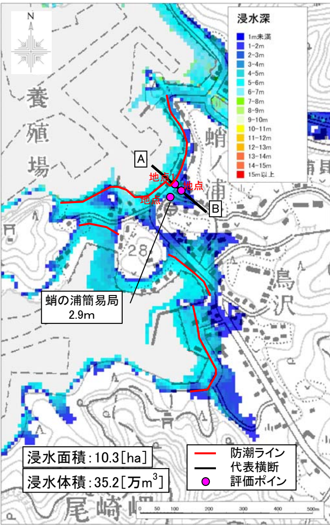
図3.4 浸水深平面分布図(施設あり)
