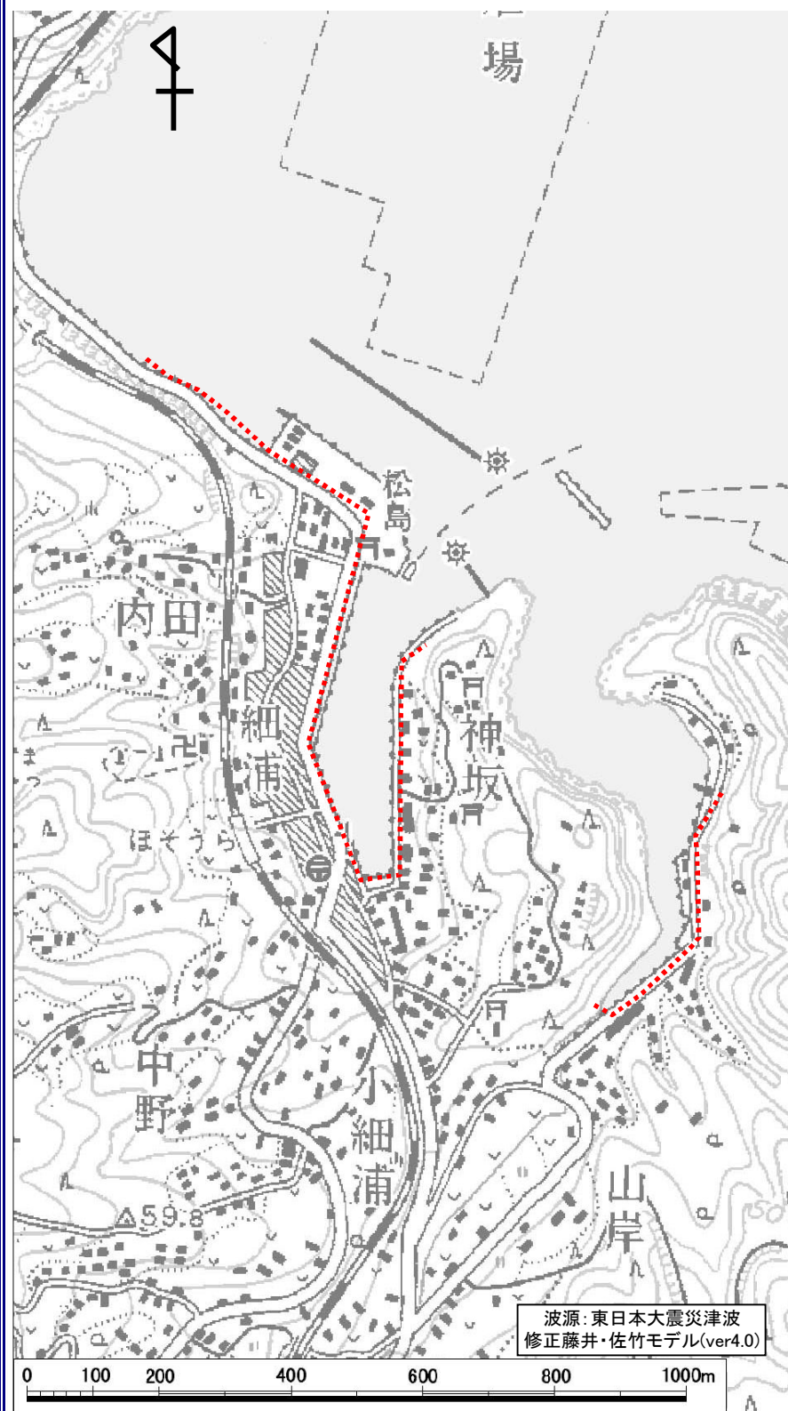
図6.15 浸水深平面分布図
