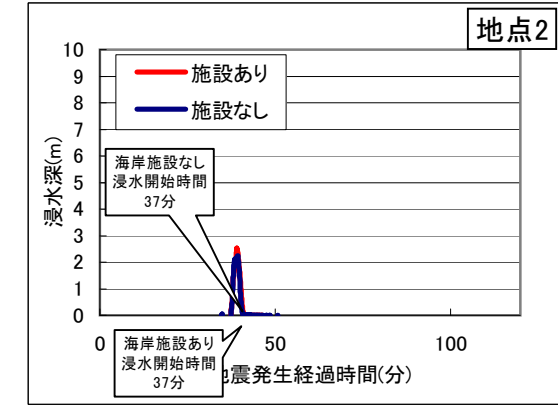
図3.7(2) 評価ポイント(堤内地)における浸水深時系列分布図
