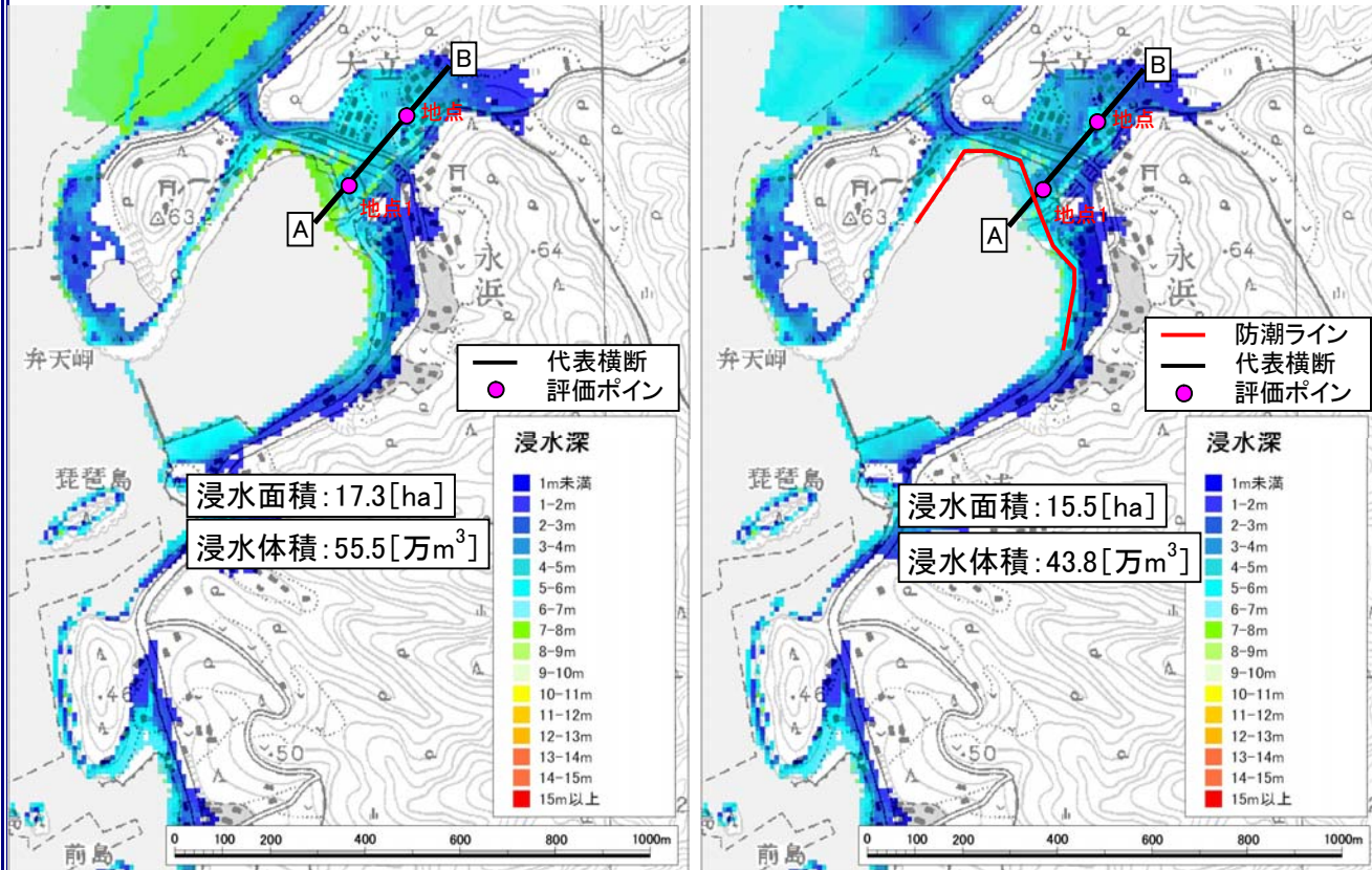
図3.13 浸水深平面分布図(施設なし)
