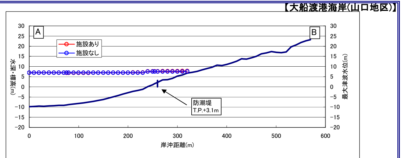
図3.20 津波最大水位
