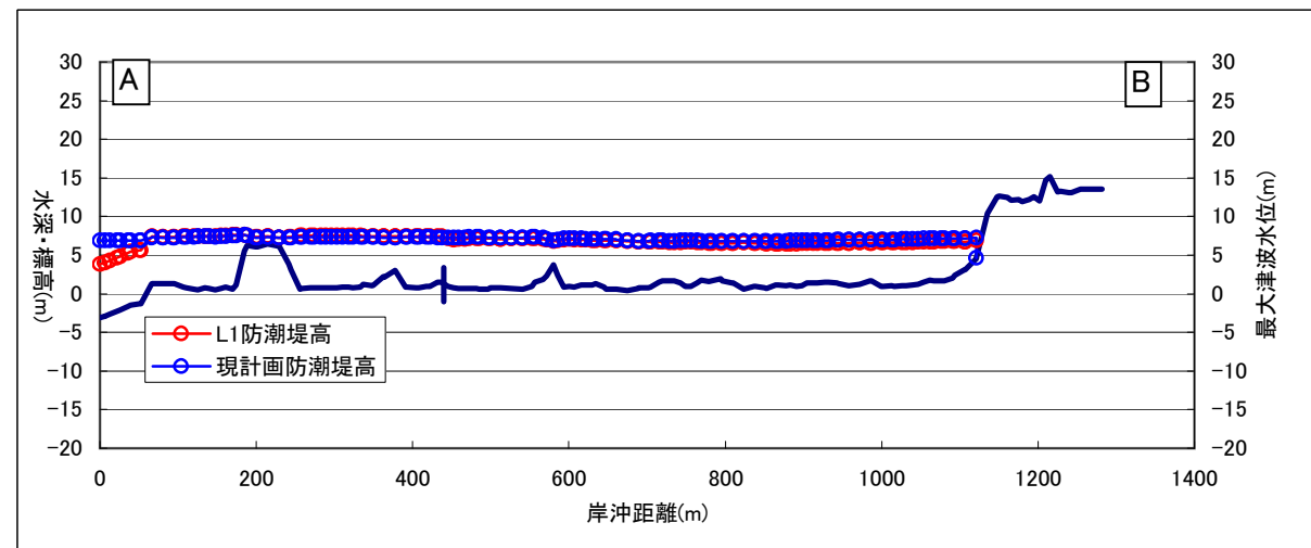
図3.26 津波最大流速
