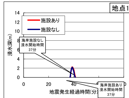
図3.12(1) 評価ポイント(防潮堤背後)における浸水深時系列分布図
