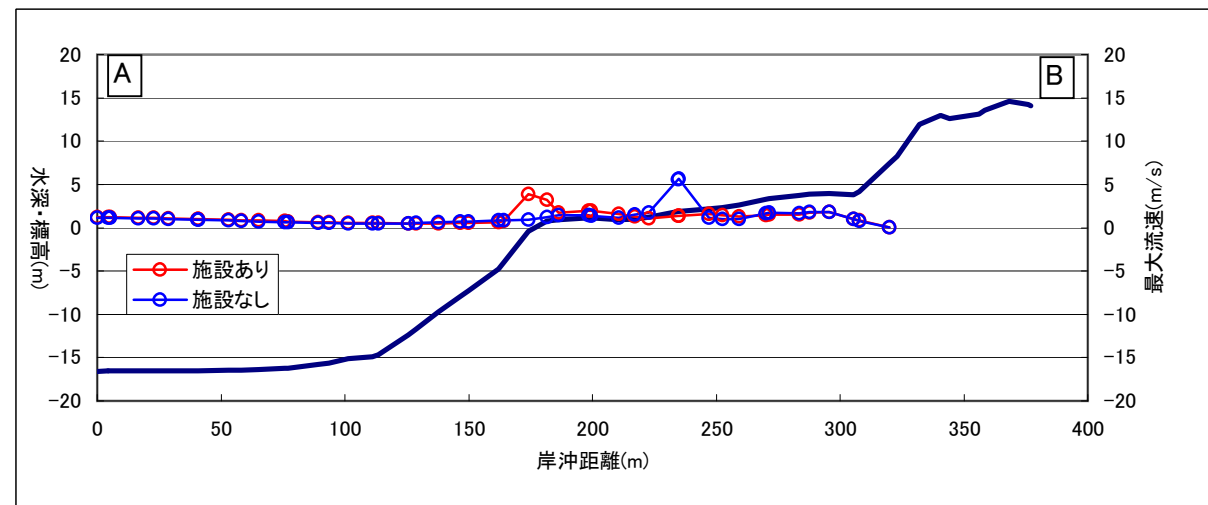
図3.6 津波最大流速
