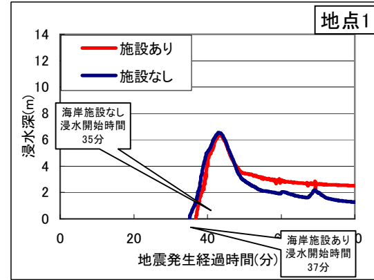
図3.27(1) 評価ポイント(防潮堤背後)における浸水深時系列分布図
