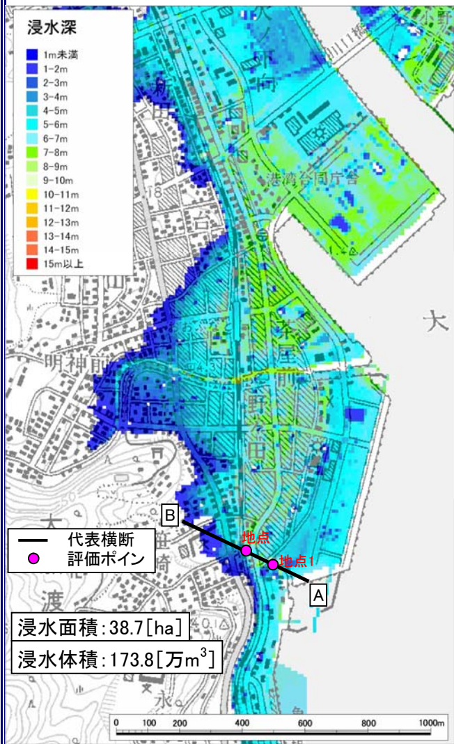
図3.28 浸水深平面分布図(施設なし)
