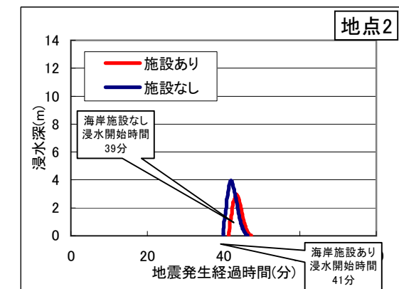
図3.17(2) 評価ポイント(堤内地)における浸水深時系列分布図
