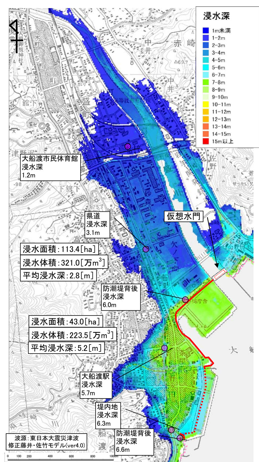
図6.11 浸水深平面分布図
