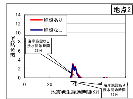
図3.38(2) 評価ポイント(堤内地)における浸水深時系列分布図
