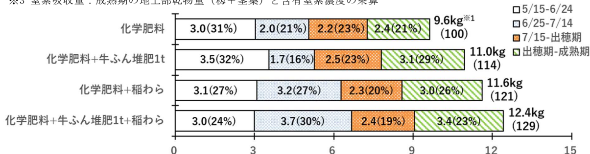
図2 水稻一作期における生育時期別窒素吸収量の内訳（kg/10a、直近 5 作平均）
