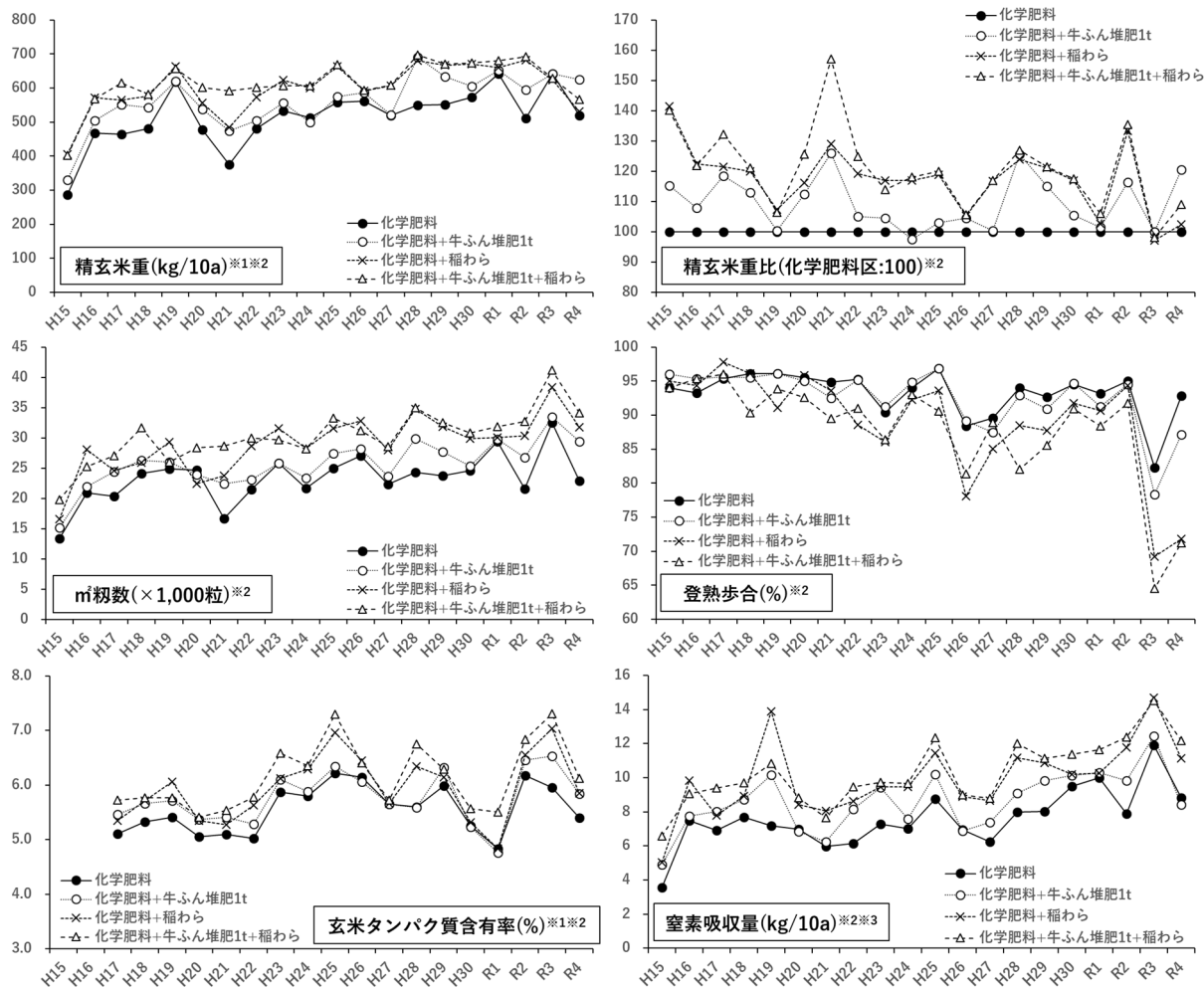
図1 水田土壌における有機物の長期連用が水稻の収量・品質等に及ぼす影響
