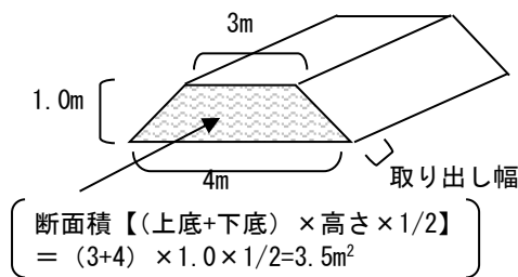
【図 1 サイロのサイズ設計例】 (例：スタックサイロの場合)
