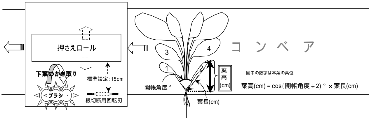
図1 ほうれんそうの葉高と調製機
