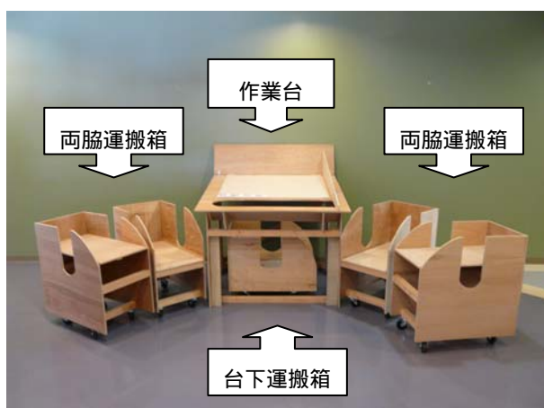
図1 りんどう選花作業台セットの構成
