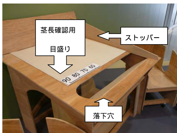
図2 りんどう選花作業台の天板の構造
