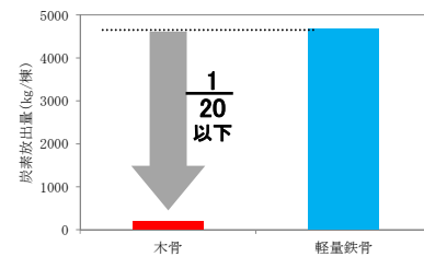
図2 資材製造時の炭素放出量 約100坪のハウス1棟に使用される骨材量から算出
