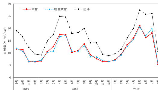
図1 平均日射量の推移 (2015.9～2017.8)
