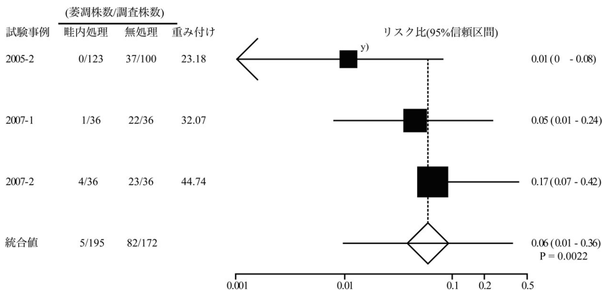
図22 クロルピクリンくん蒸剤マルチ畦内処理（消毒畦幅90 cm）の萎凋株発生抑制効果 2)
