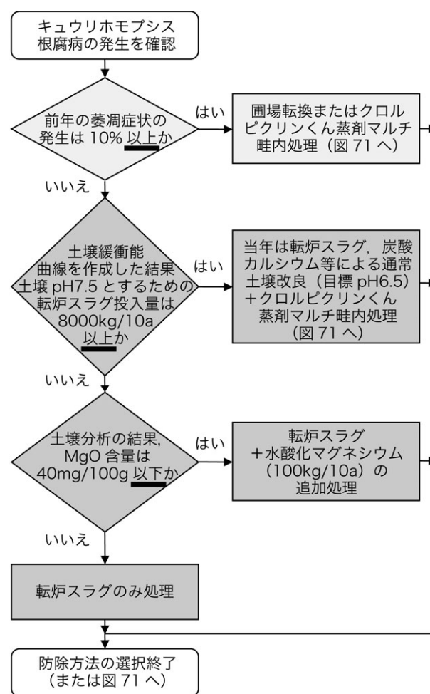
図 79 転炉スラグを用いた土壤 pH 改良による被害軽減技術選択のフローチャート
