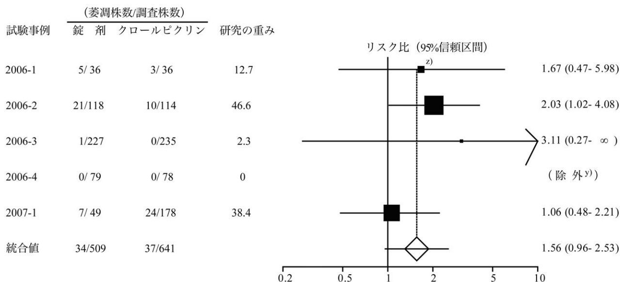
図44 クロールピクリン錠剤によるキュウリモブシス根腐病の萎凋株発生抑制効果
