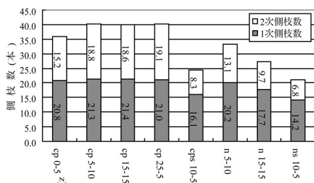
図27 定植59日後 (8月5日) 側枝数調査結果 (2005) z)試験区の構成は「表25」のとおり。
