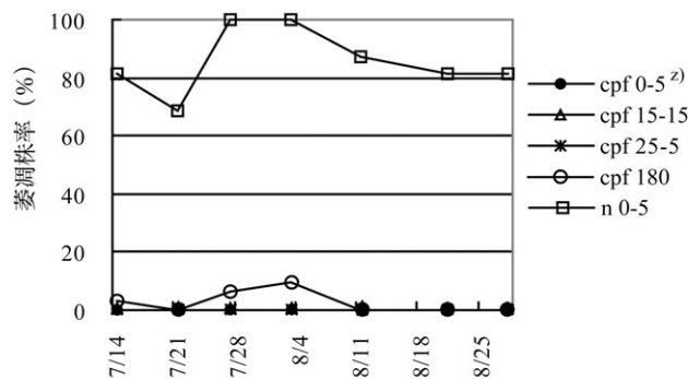
図36 萎凋株の発生推移（2006，試験反復Ⅱ） z)試験区の構成は‘表26’のとおり。
