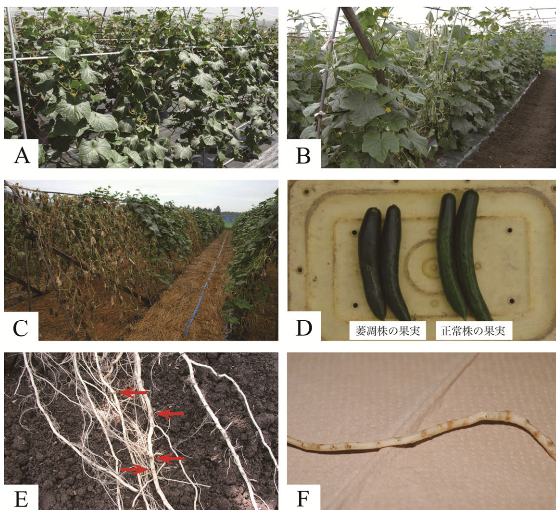
図 1 岩手県の露地夏秋作型キュウリにおいて観察された病徴 (1)
