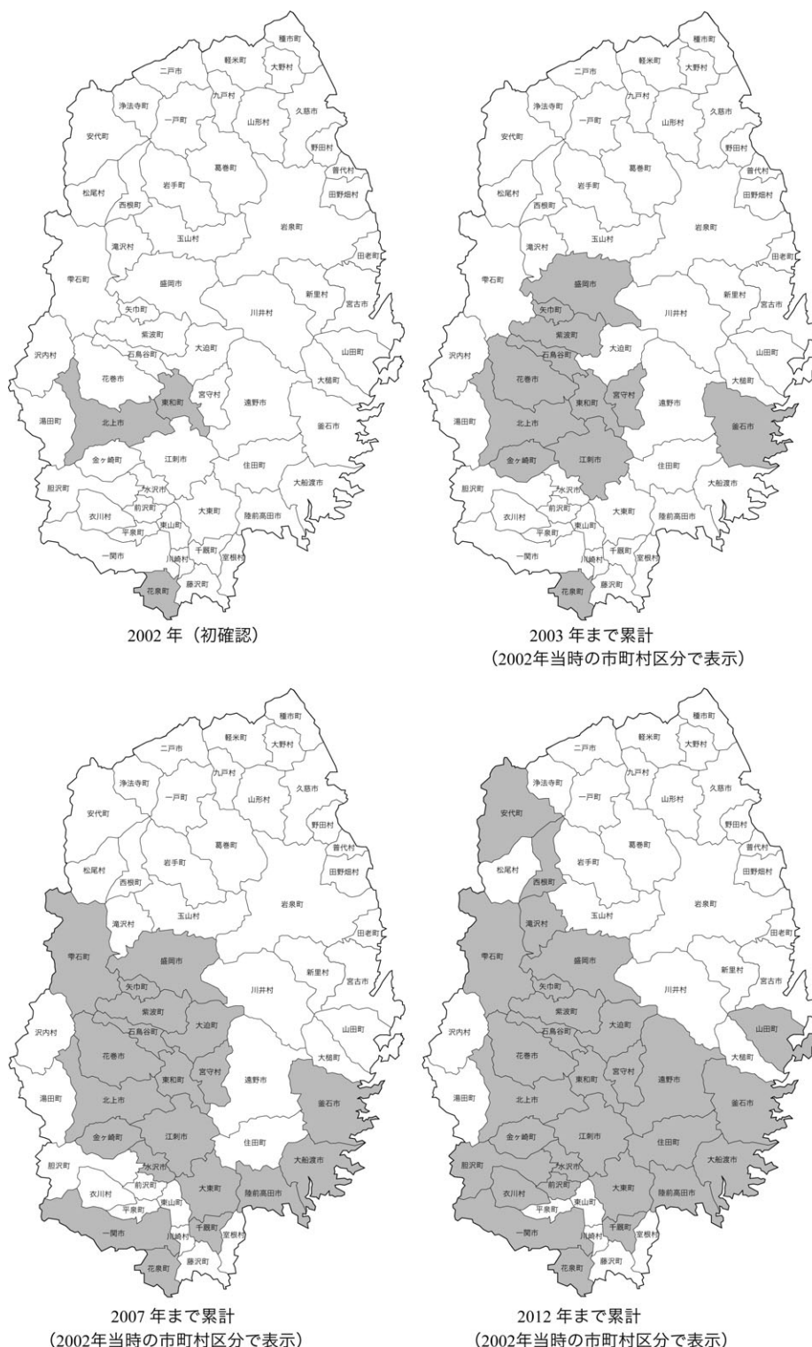
図5 岩手県におけるキュウリホモブシス根腐病の発生確認地域の変遷
