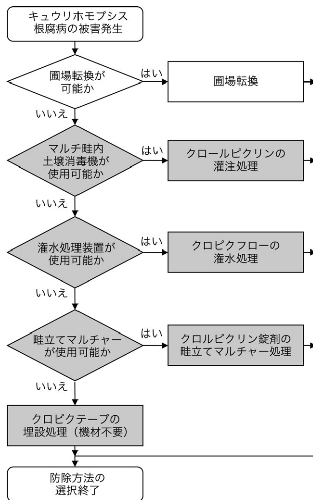
図71 クロルピクリンくん蒸剤マルチ畦内処理における剤型選択のフローチャート
