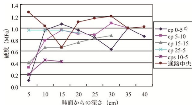
図32 各試験区における土壌硬度 (2005)
