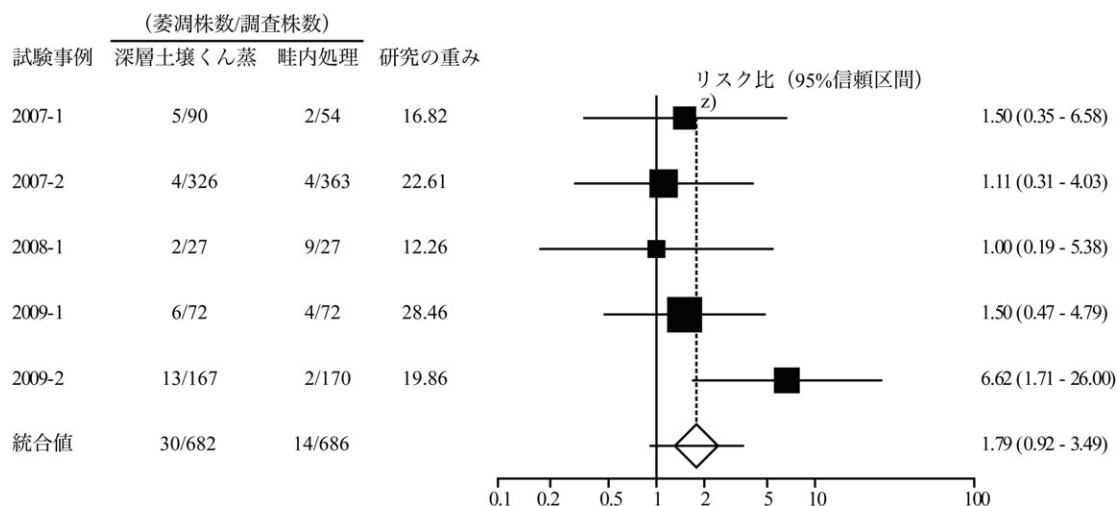
図47 クロルピクリンくん蒸剤を用いた深層土壌くん蒸処理とマルチ畦内処理の萎凋株発生抑制効果の比較
