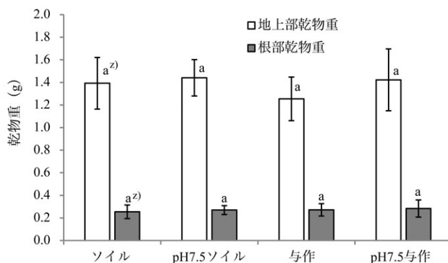
図55 各種育苗培土で栽培したキュウリ苗の地上部および根部乾物重 (キュウリ播種35日後)
