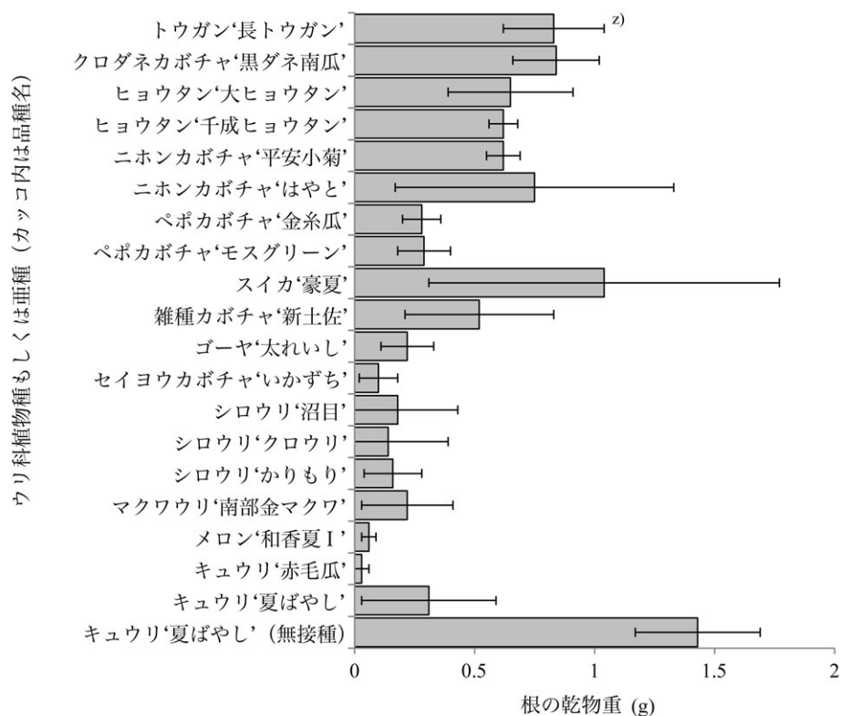
図 19 ホモブシス根腐病抵抗性検定試験におけるウリ科植物種・亜種の根乾物重の差異 z) エラーバーは標準偏差を示す。
