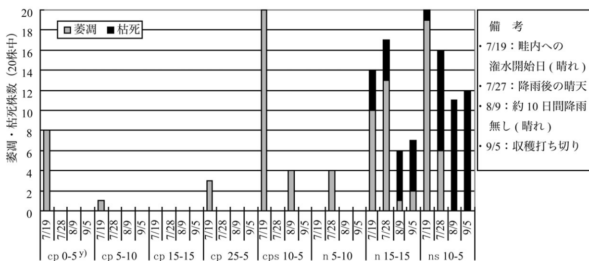
図30 試験区における萎凋・枯死株の発生推移 (2005) z) z)汚染程度の高い反復Ⅱでの結果, y)試験区の構成は‘表25’のとおり.
