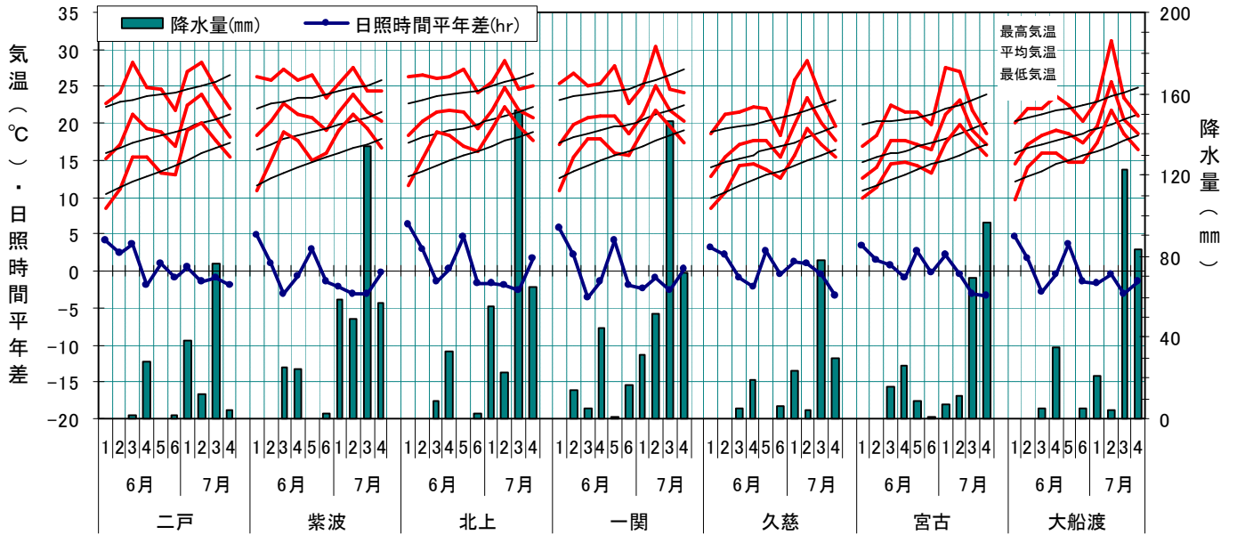
図1 半旬別気象経過（アメダス地点、6月第1半旬～7月第4半旬）
