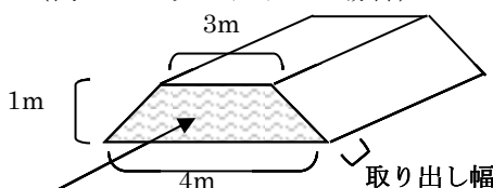
【図2 サイロのサイズ設計例】
