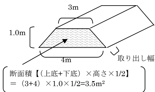
【図2 サイロのサイズ設計例】 (例：スタックサイロの場合)
