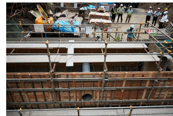
被災木を活用した治山ダム工事の残存型枠 （岩手県）
