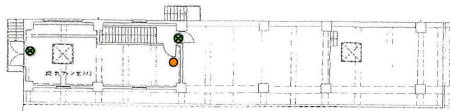
— 16 平面図 1:100
