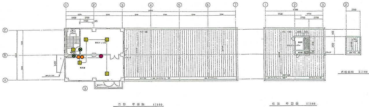
二階平面図 1:100
