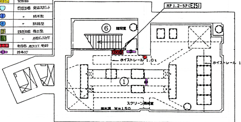
地下3階 平面図 1/100
