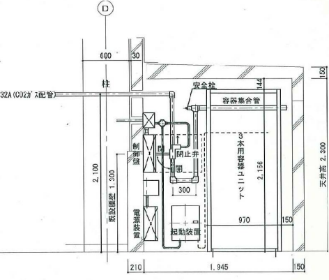
北面 展開図 (B-B断面)
