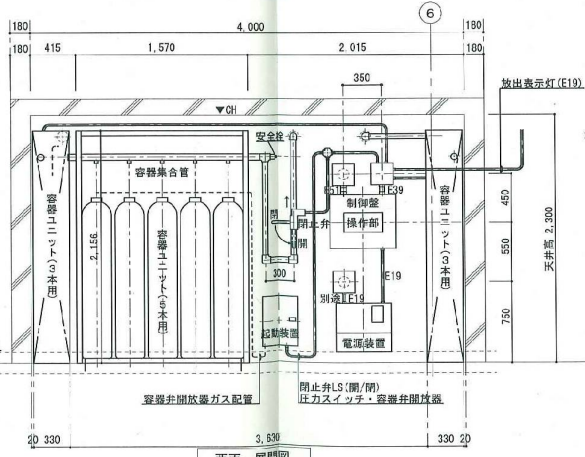
西面 展開図
