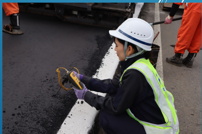
舗装初期締固め温度の測定
