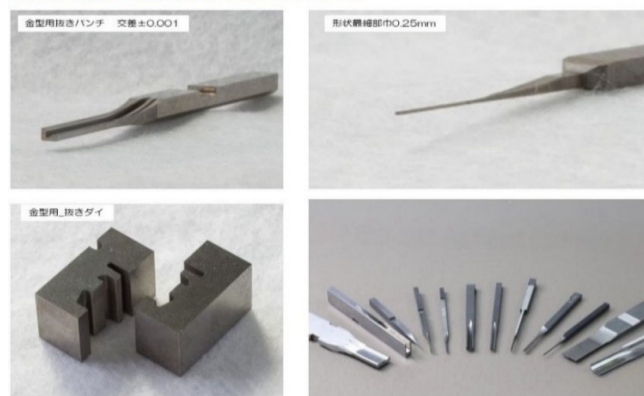
■微細な微細研削加工（プロファイルグラインダー）
