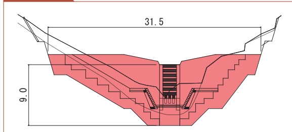
側面図
