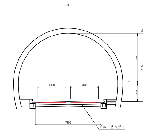
標準横断面図（つなぎトンネル） S=1:50
