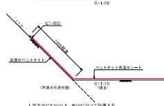
地山との接続図
