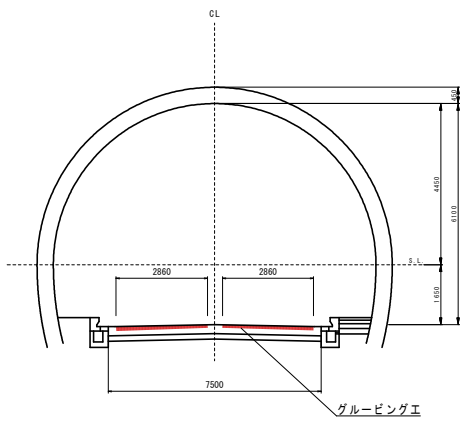
標準横断面図（深戸トンネル） S=1:50
