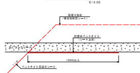
構造物底面接続図
