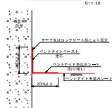
構造物側面接続図
