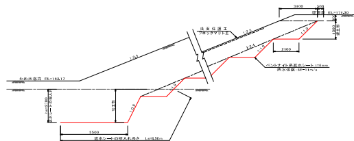
構造物側面接続図
