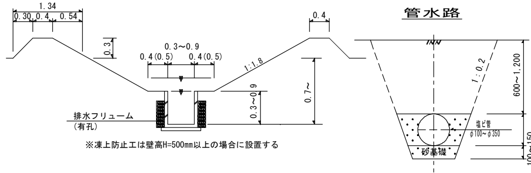
小排水路
