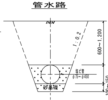
用水路工
