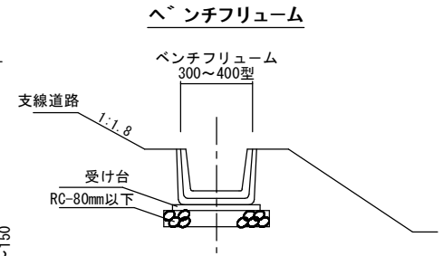
用水路工
