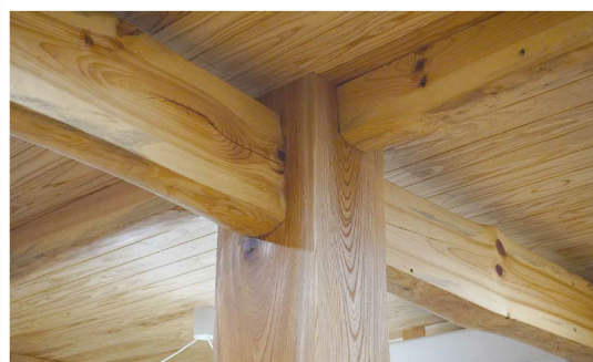
談話・学習スペースの荷重を支える恵比寿柱
