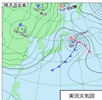
3月6日09時
