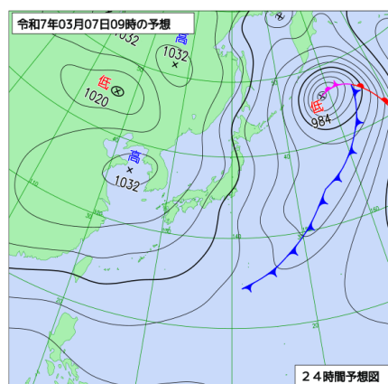
3月7日09時予想
