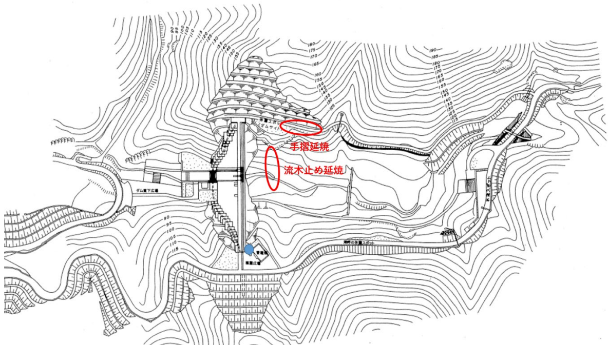
綾里川ダム平面図
