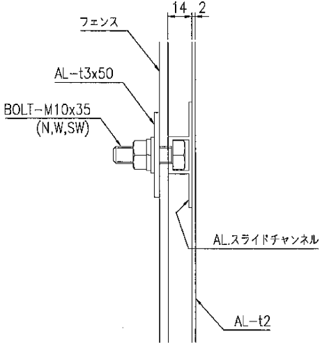
取付部詳細図 S=1/2
