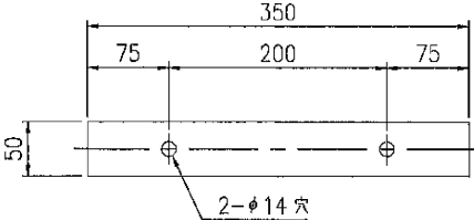
AL-t3x50 詳細図 S=1/5
