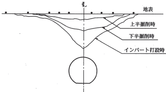
図 6-13 地中沈下分布 (横断方向)
