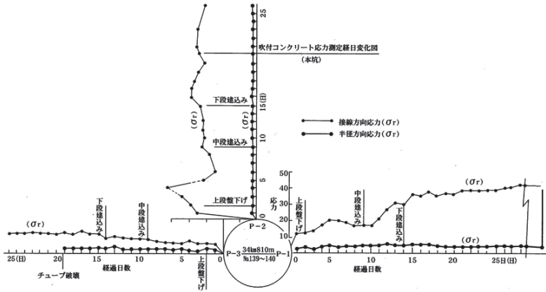
図 6-6 吹付コンクリート応力分布図
