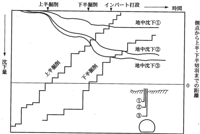
図 6-12 地表沈下量経時変化
