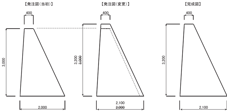
図 6-1 発注図と完成図の関係
