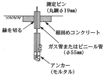
図 6-8 地中沈下測定点 of 設置例
