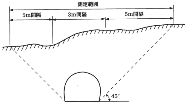
図 6-7 地表沈下の測定範囲及び間隔
