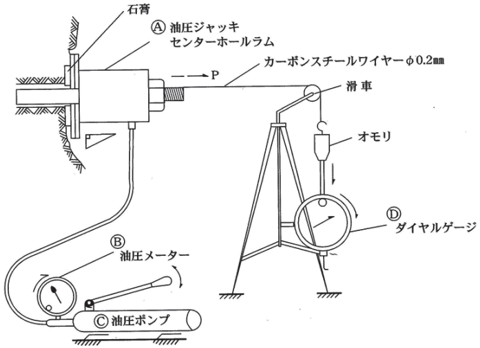
図 4-3 引抜試験概要図
