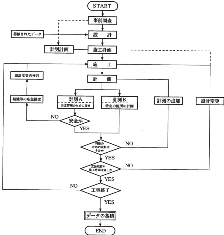
図 4-1 計測フロー
