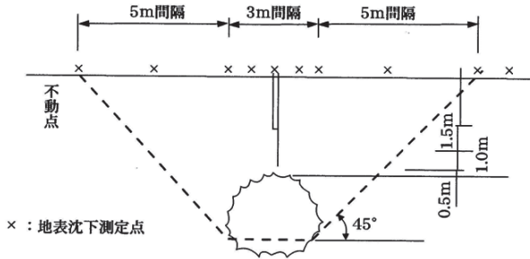
図 6-9 地中沈下測定点の設置例
