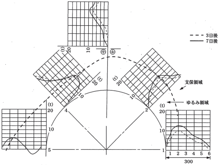
図 6-3 ロックボルトの軸力分布
