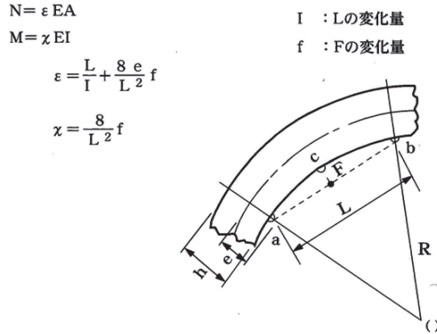
図6-5 コバリーの図
