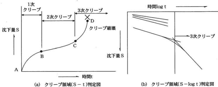
図5-1 天端沈下のクリープ領域判定図
