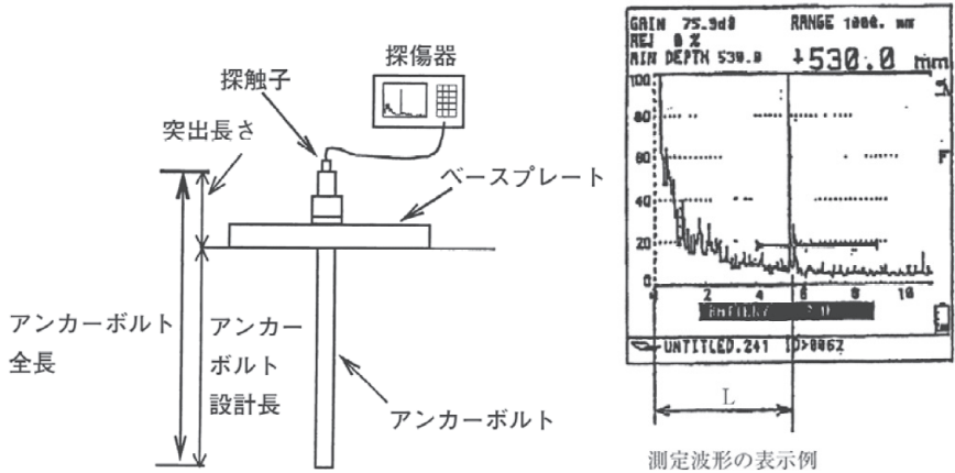
アンカーボルト長さの測定の例
