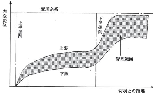
図5-4 内空変位管理図の例
