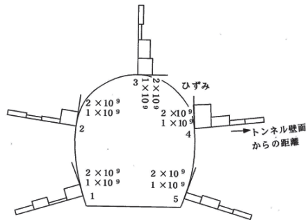
図6-2 地中ひずみ分布
