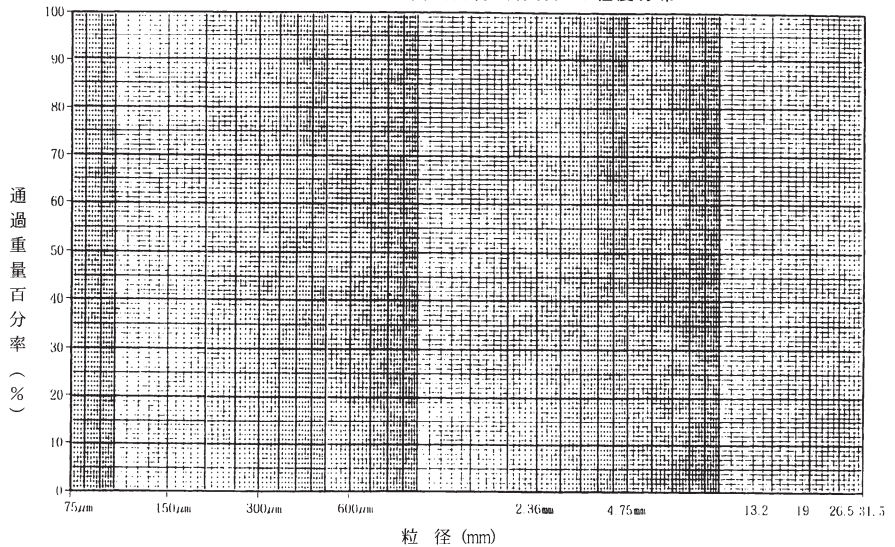
アスファルト抽出残留物（骨材）の粒度分布
