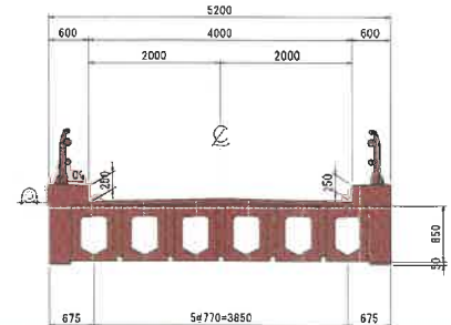
上部工断面図
