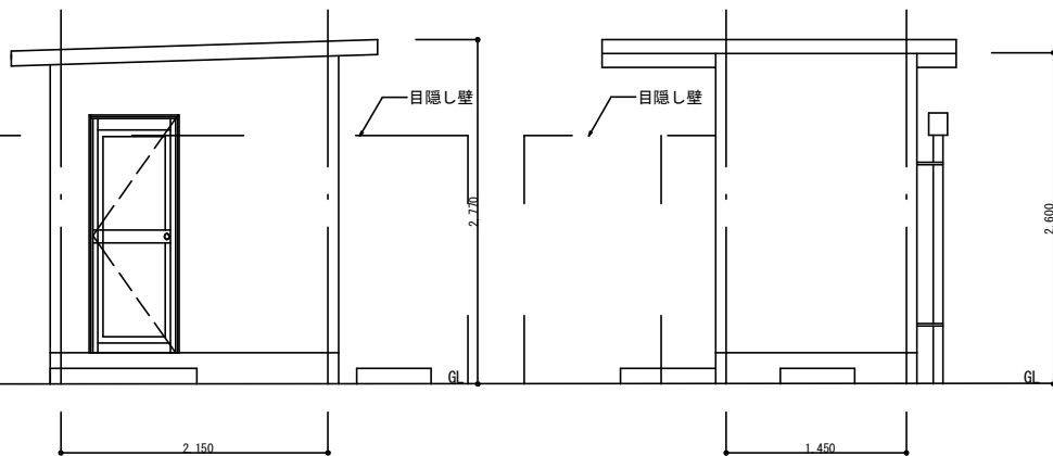
北立面図 1/25
