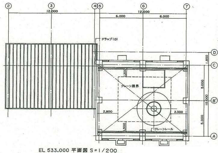
EL 533.000 平面図 S=1/200
