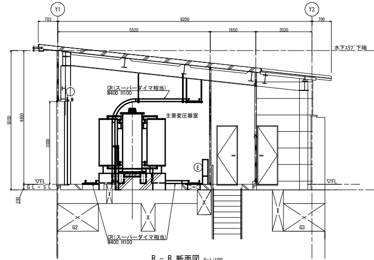
B - B 断面図 S=1/100
