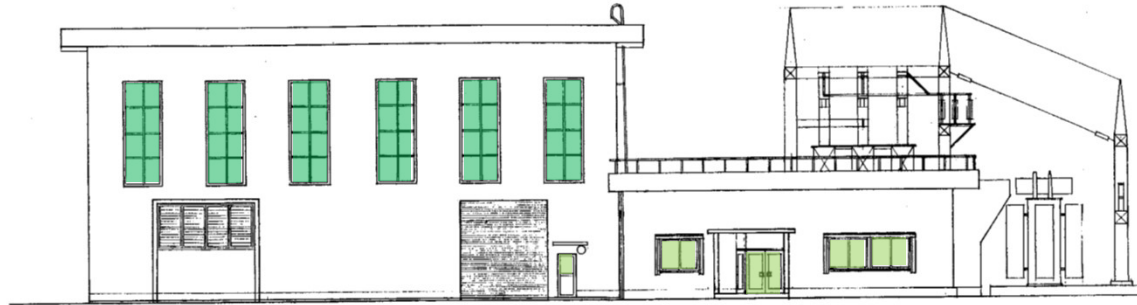
南立面図
