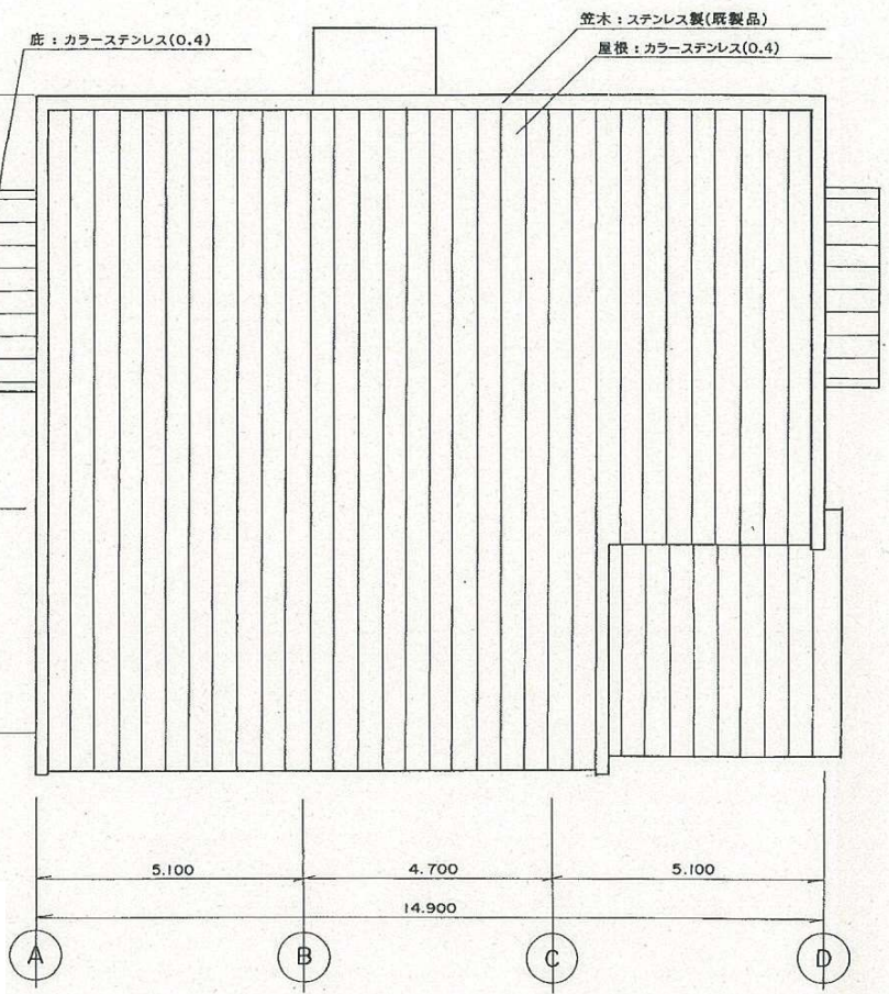
屋根 平面図 S=1/100
