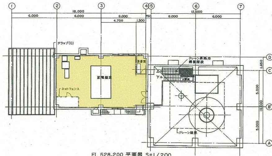
EL 528.200 平面図 S=1/200
