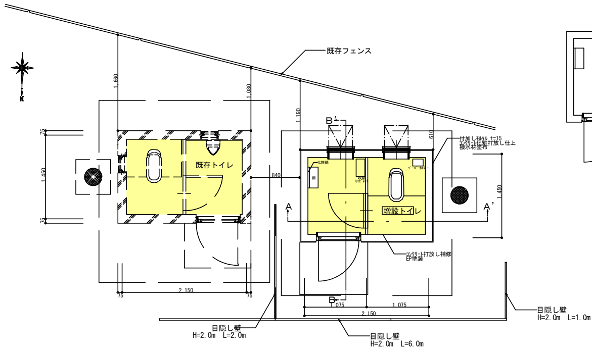
配置兼平面図 1/25
