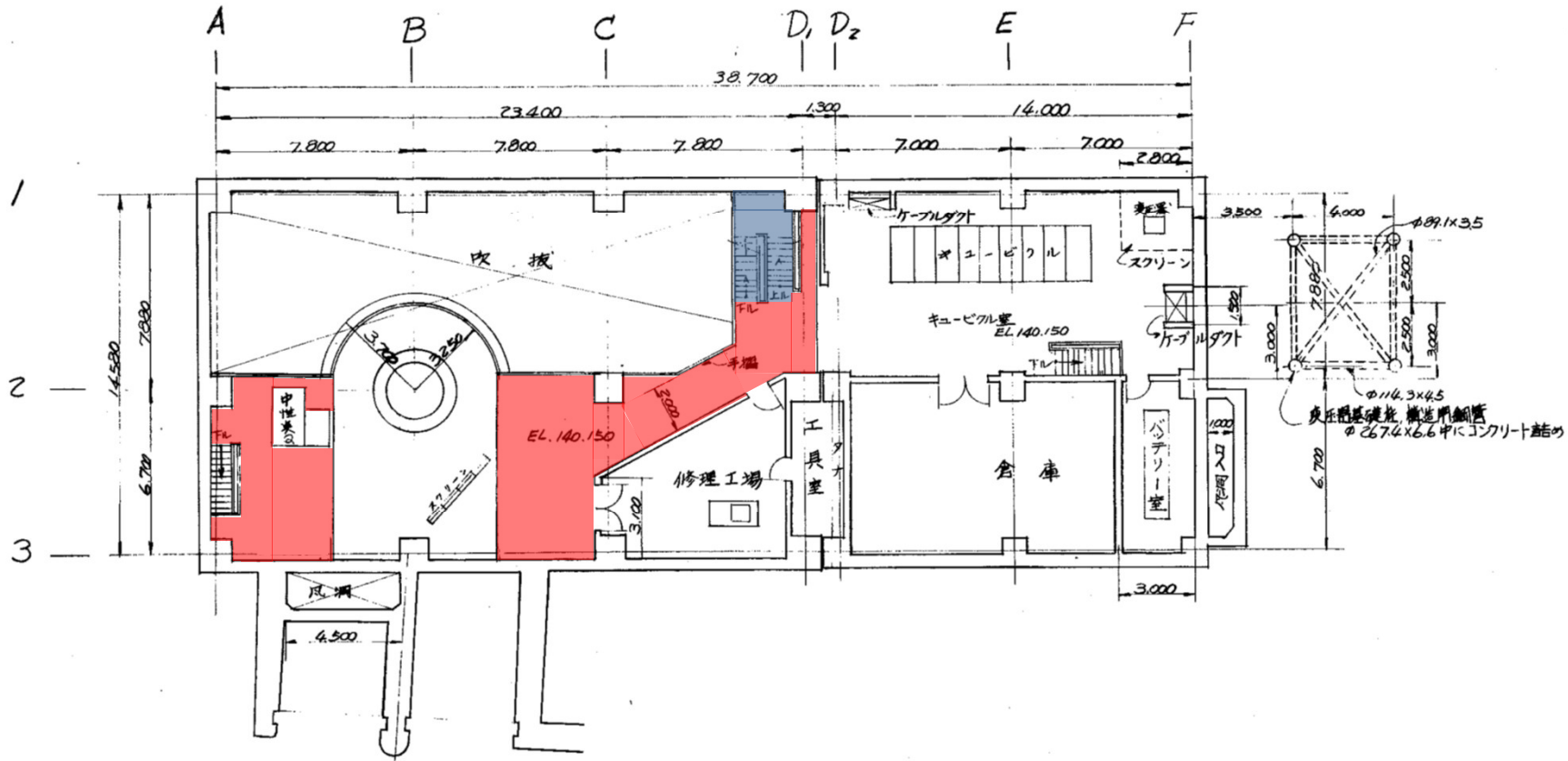
EL.140.150 平面図 (地下1階)
