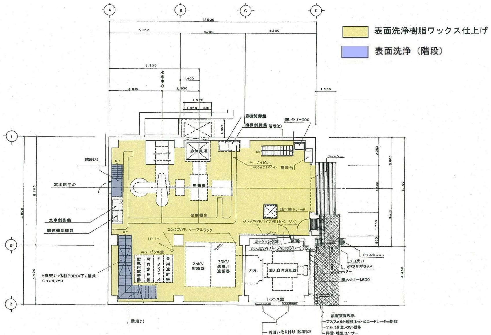
1階平面図 EL. 731.500
