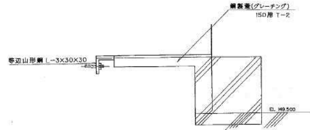
流し管布設詳細図 S=1/40
