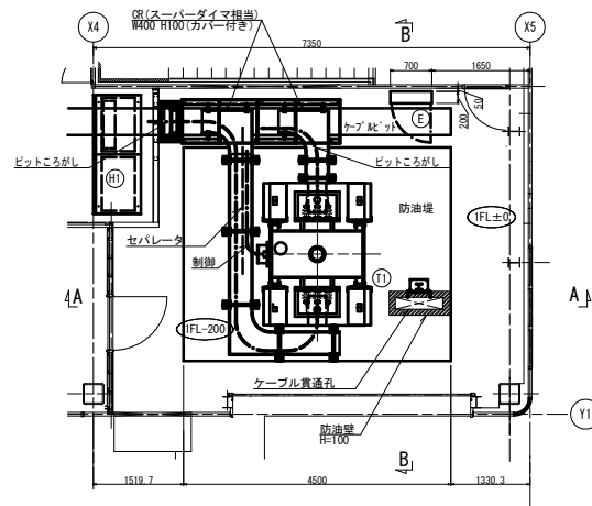
ケーブル配線概要図 S=1/100
