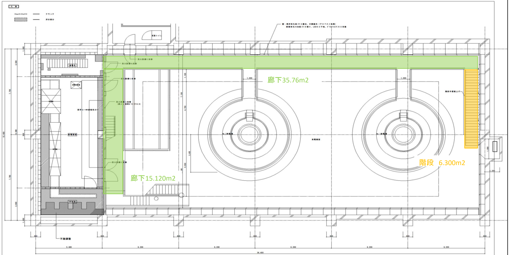
配電盤室他 平面図 S=1/50 (E.L. 269.400)
