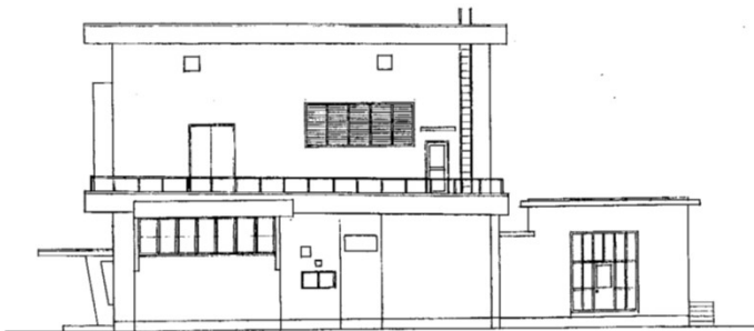
東立面図
