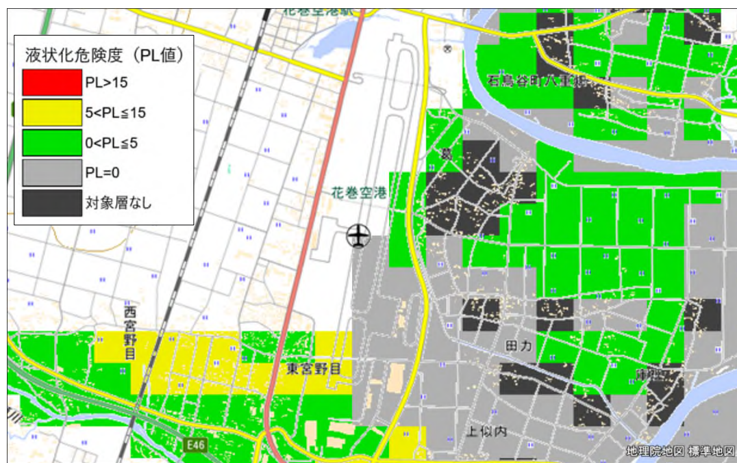
図 3.3.3-10 日本海溝（三陸・日高沖）モデルによる空港周辺の液状化危険度
