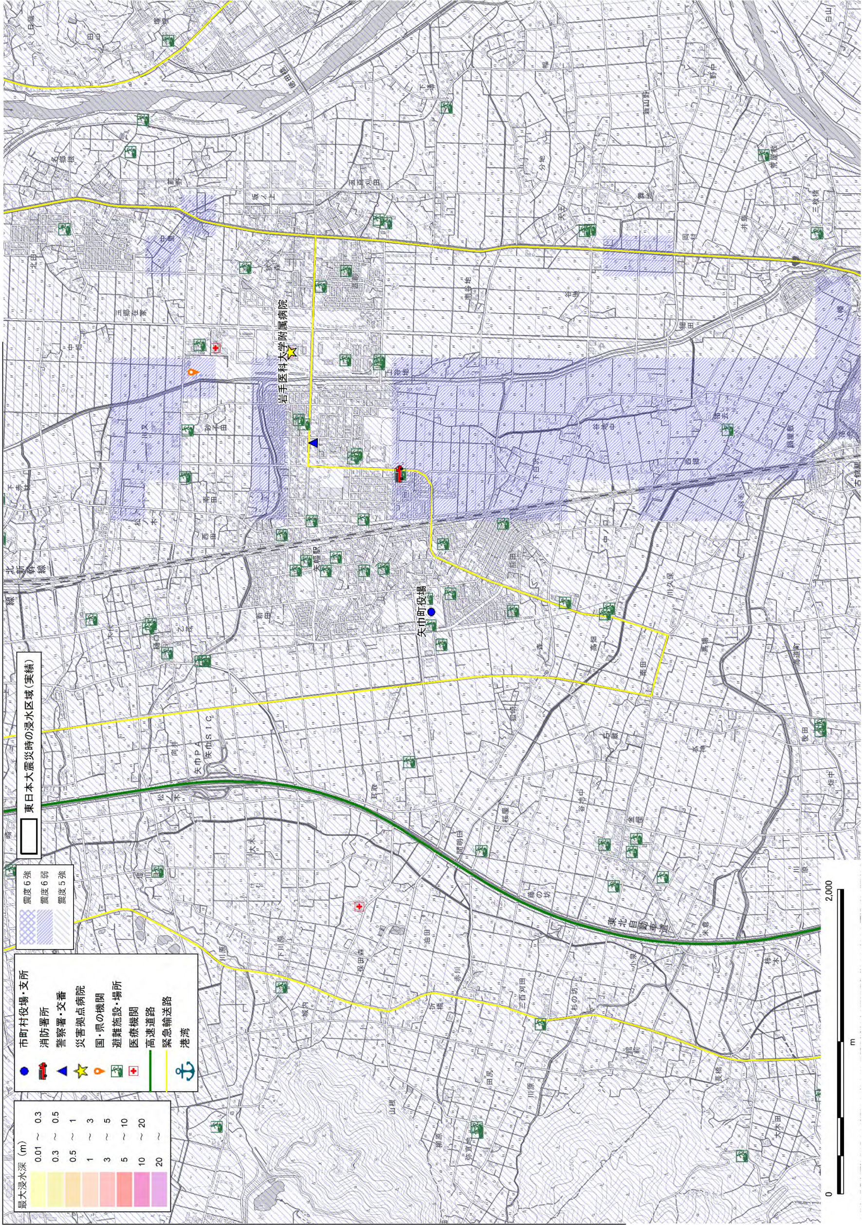
図 3. 4. 1-38 震度分布と防災上の重要施設の重ね合わせ図 (矢巾町)
