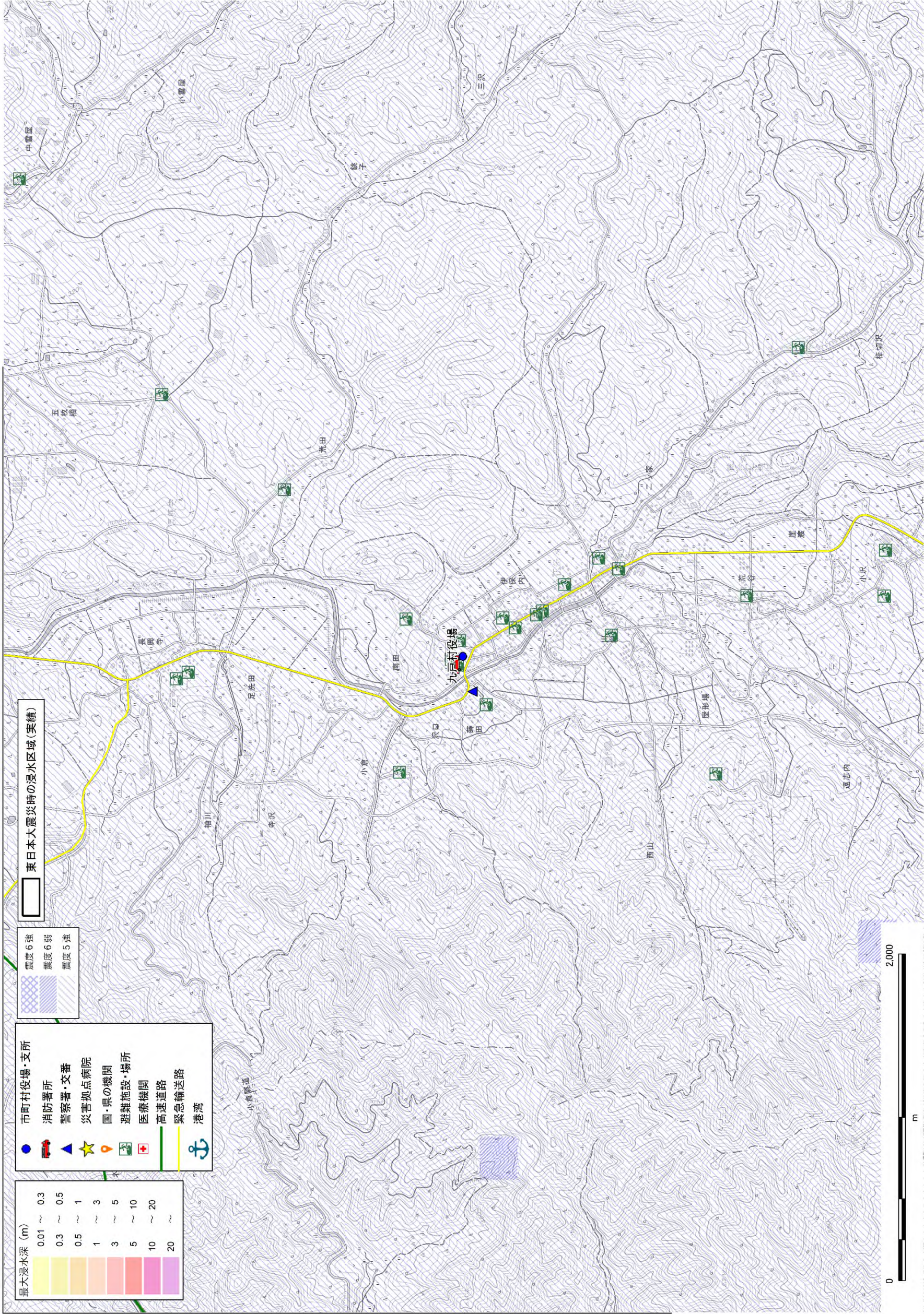
図 3.4.1-44 震度分布と防災上の重要施設の重ね合わせ図 (九戸村)
