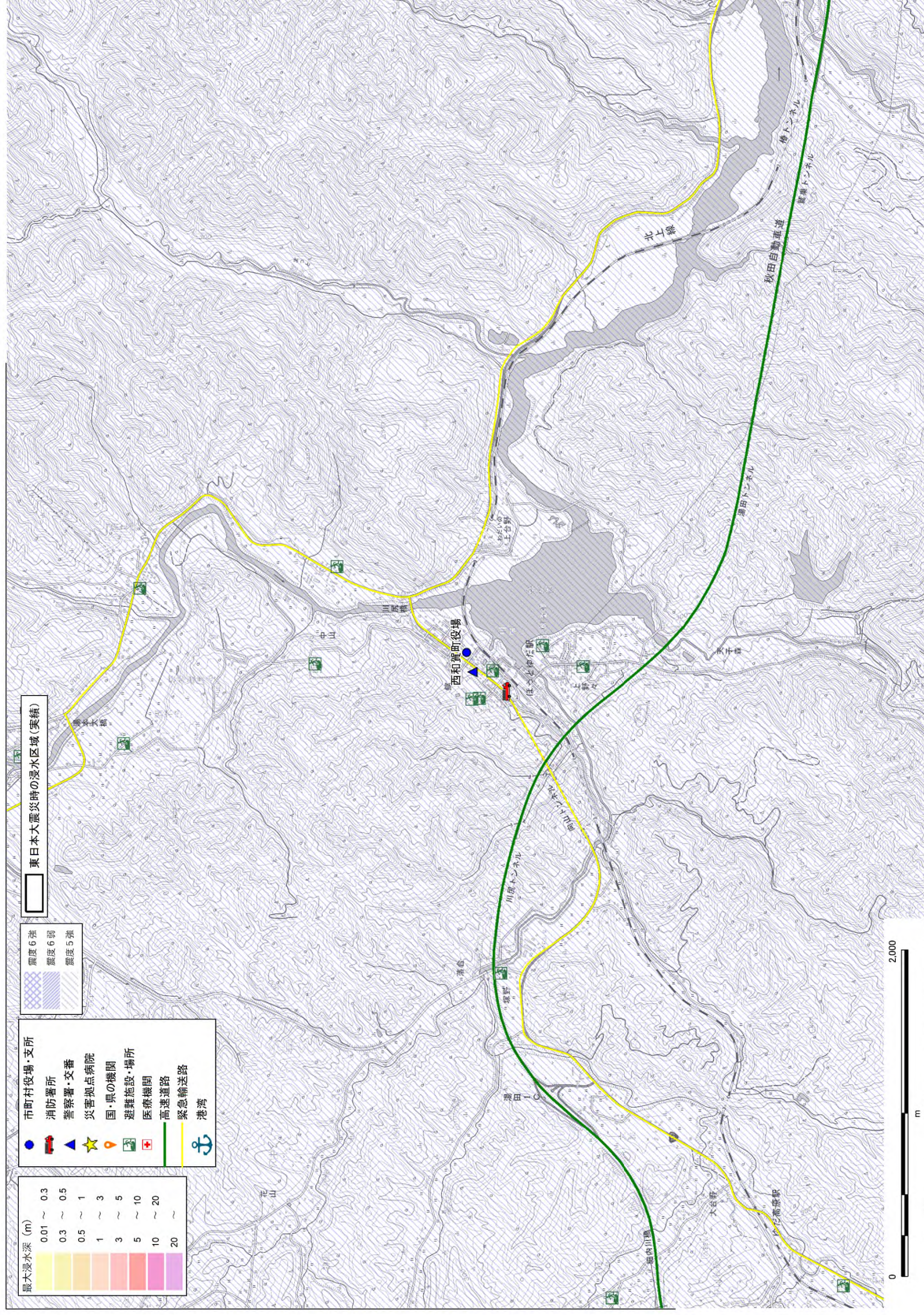
図 3.4.1-39 震度分布と防災上の重要施設の重ね合わせ図 (西和賀町)
