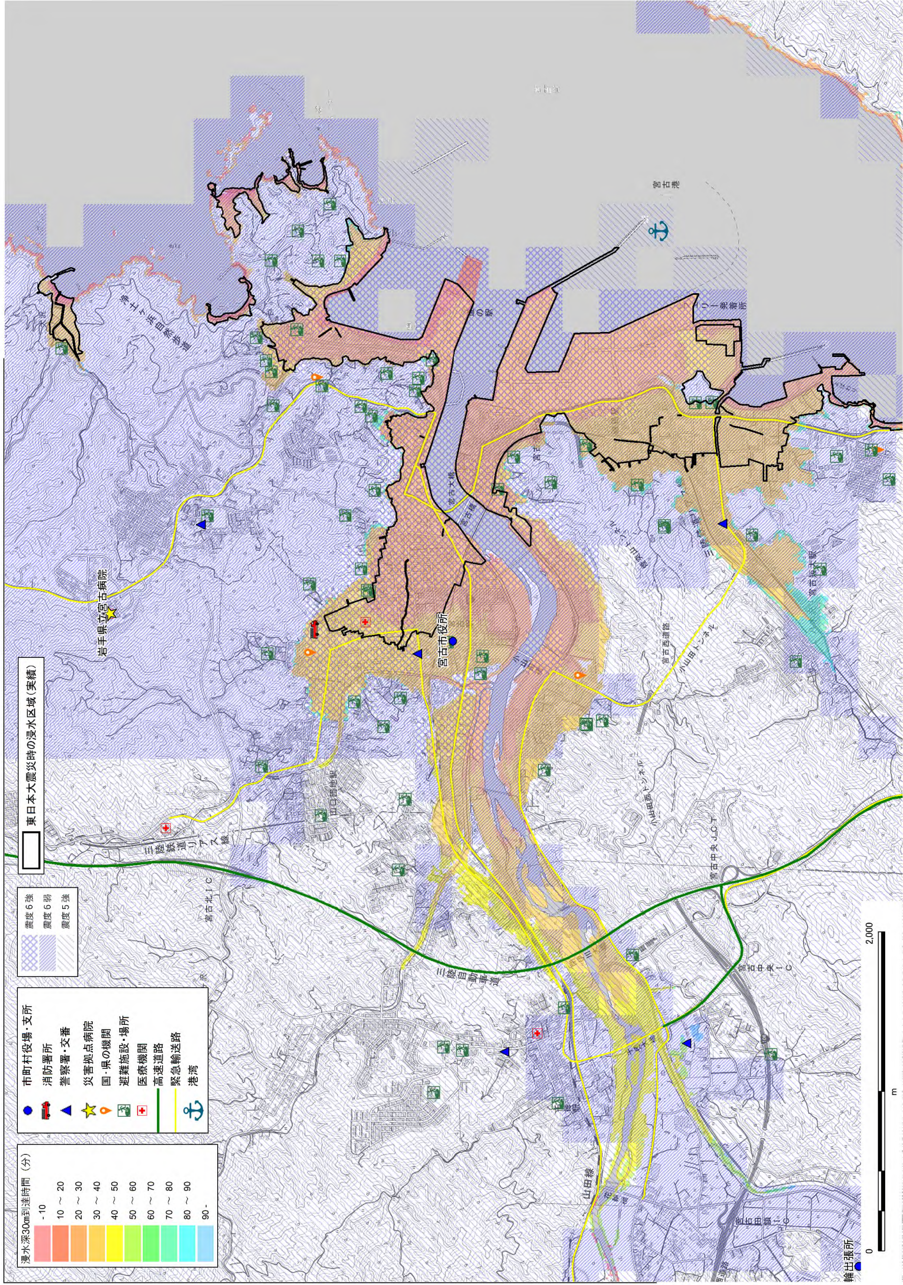
図 3. 4. 1-14 津波 30cm 到達時間・震度分布と防災上の重要施設の重ね合わせ図 (宮古市)
