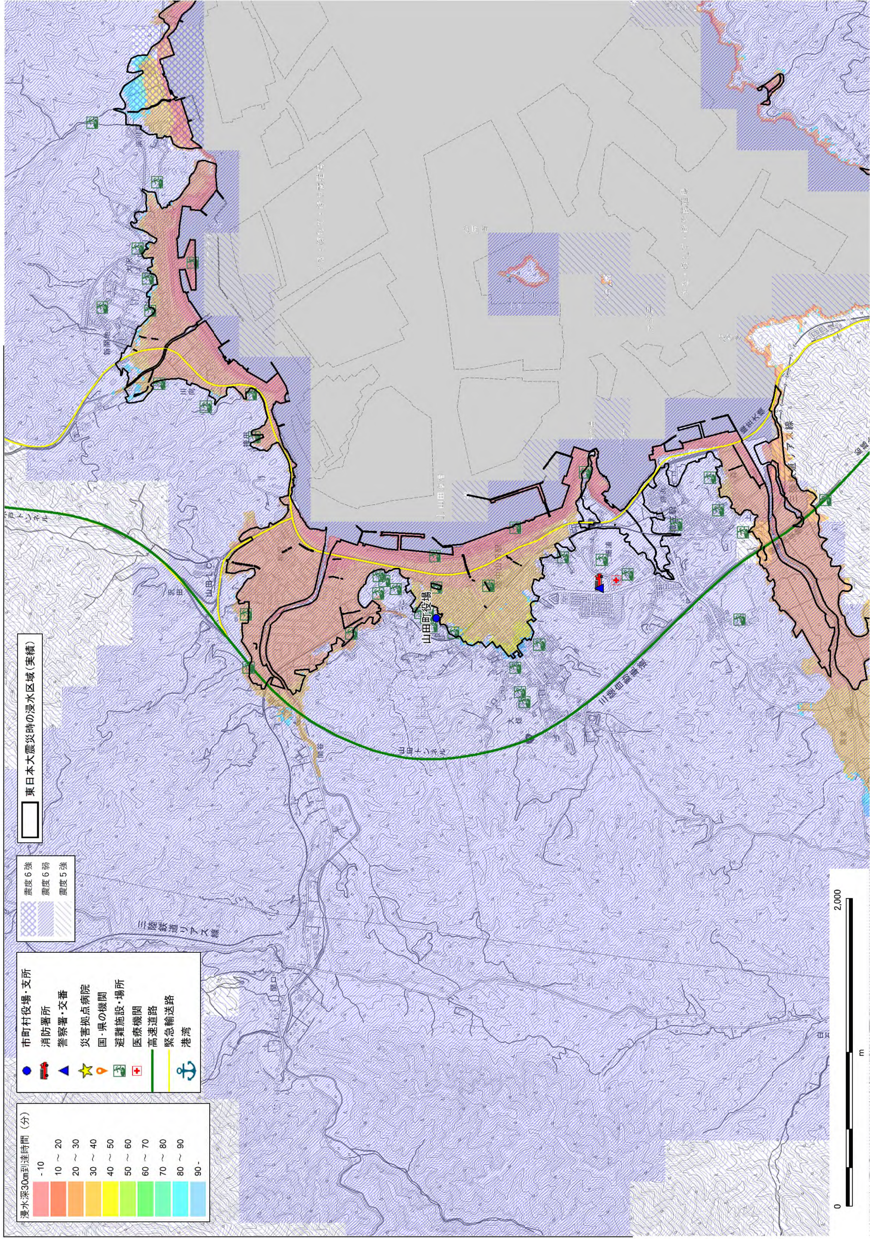
図 3. 4. 1-16 津波 30cm 到達時間・震度分布と防災上の重要施設の重ね合わせ図（山田町）
