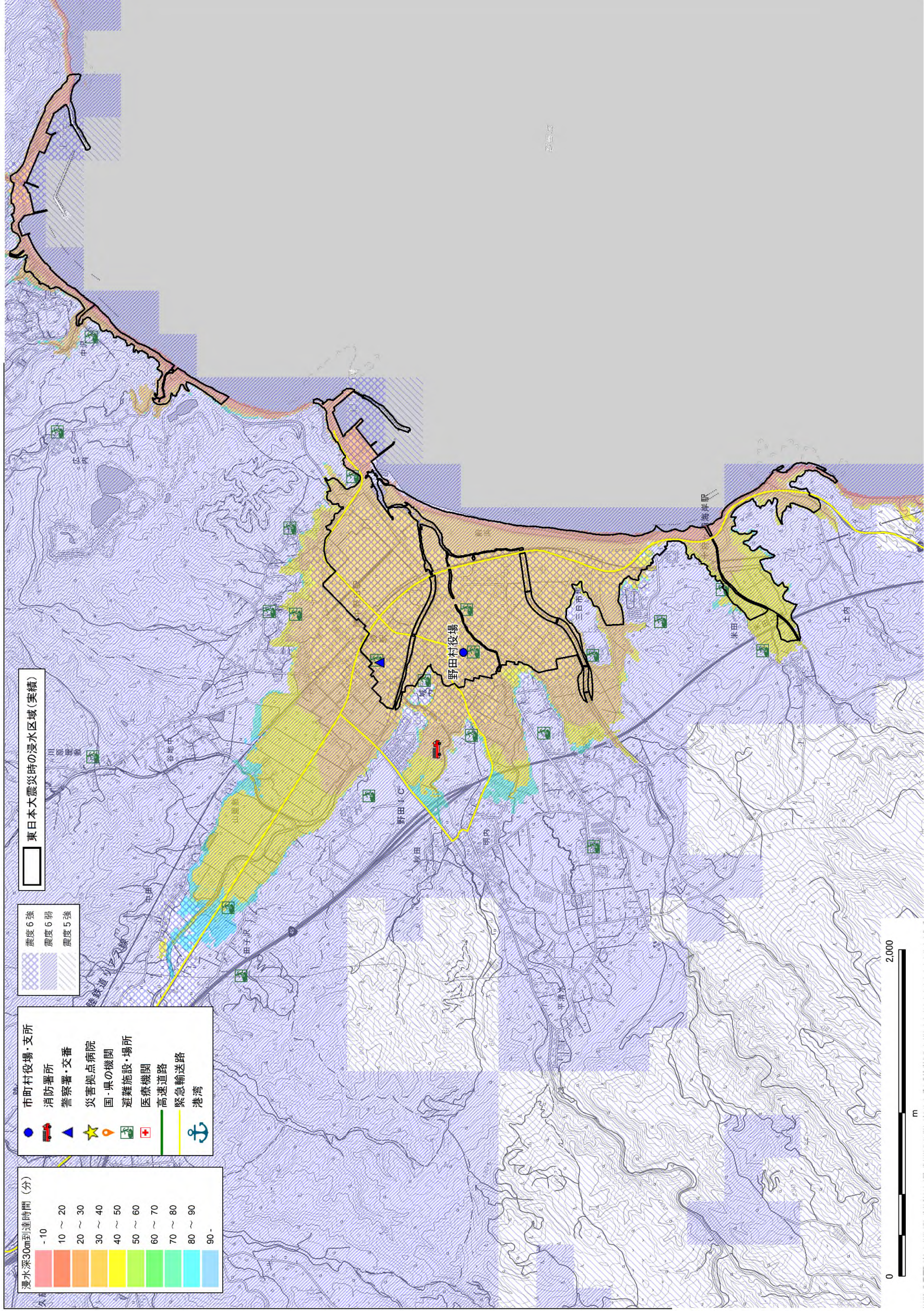
図 3.4.1-6 津波 30cm 到達時間・震度分布と防災上の重要施設の重ね合わせ図(野田村)
