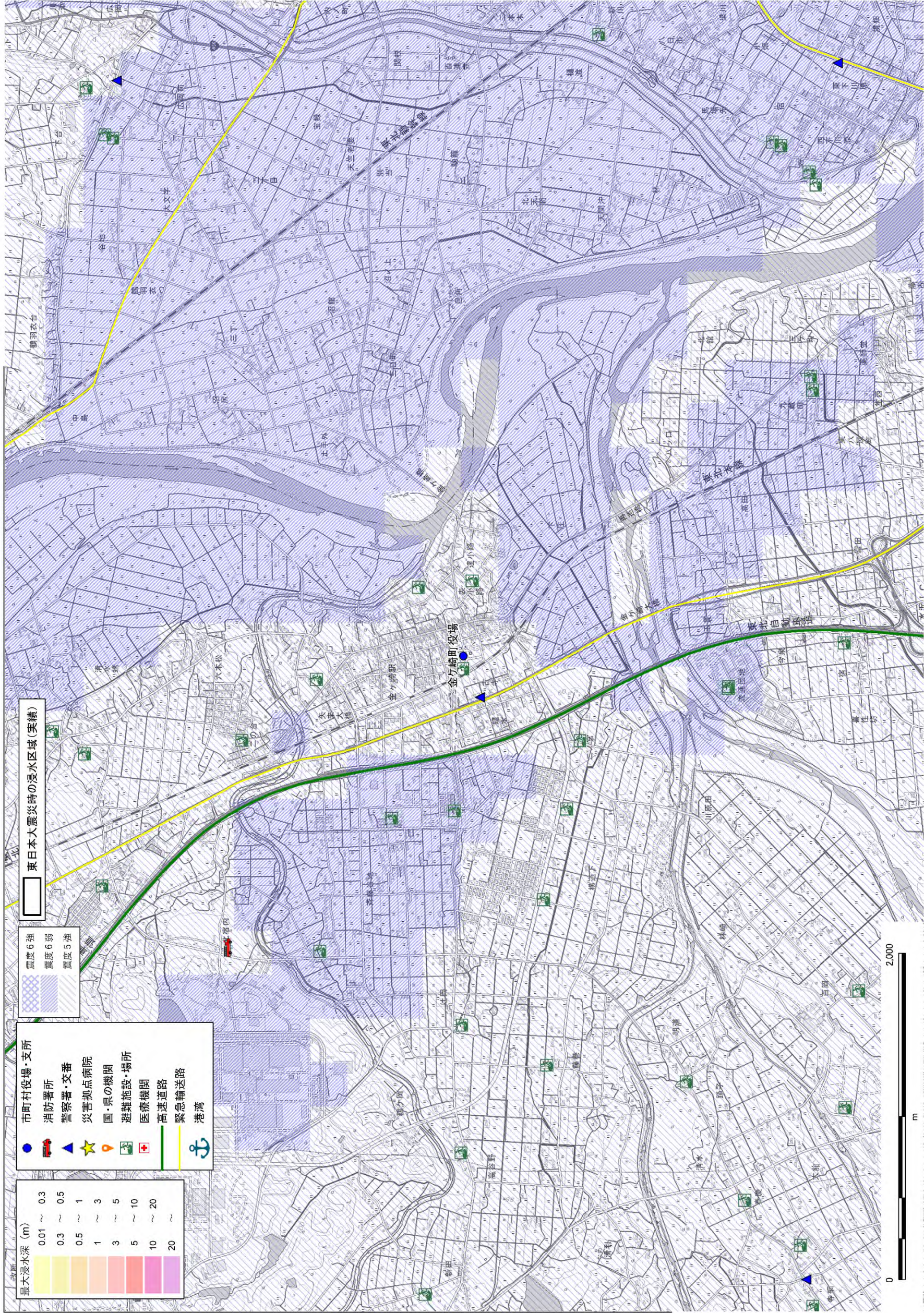
図 3. 4. 1-40 震度分布と防災上の重要施設の重ね合わせ図 (金ヶ崎町)
