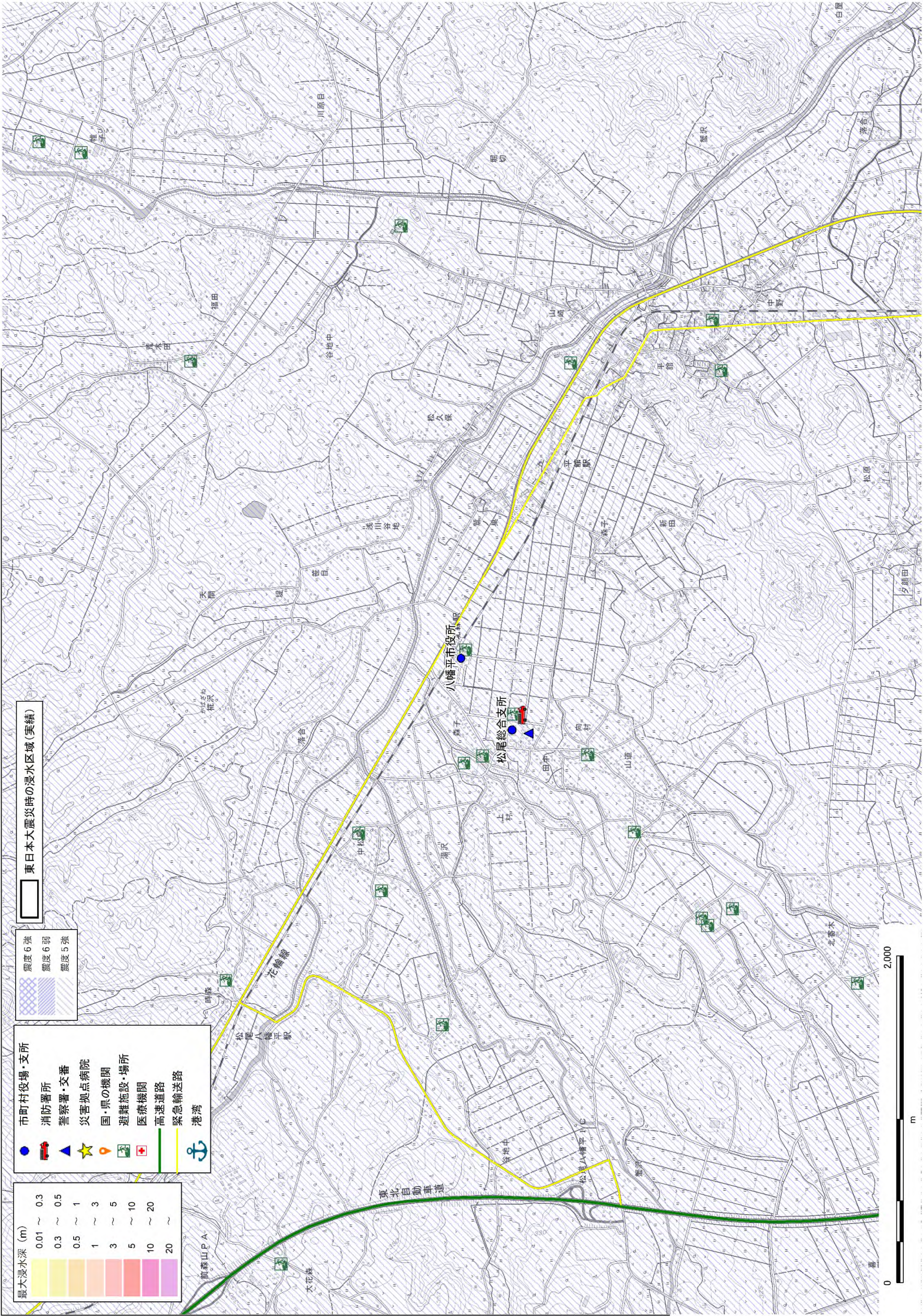
図 3. 4. 1-31 震度分布と防災上の重要施設の重ね合わせ図（八幡平市）
