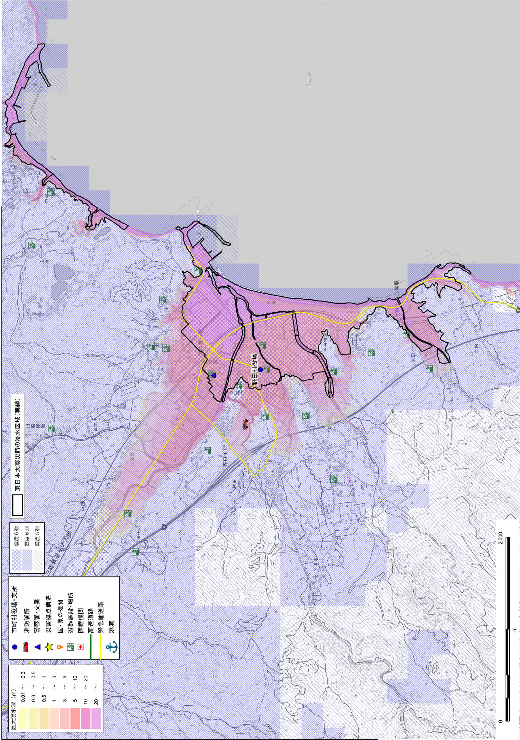
図 3.4.1-5 浸水深・震度分布と防災上の重要施設の重ね合わせ図（野田村）
