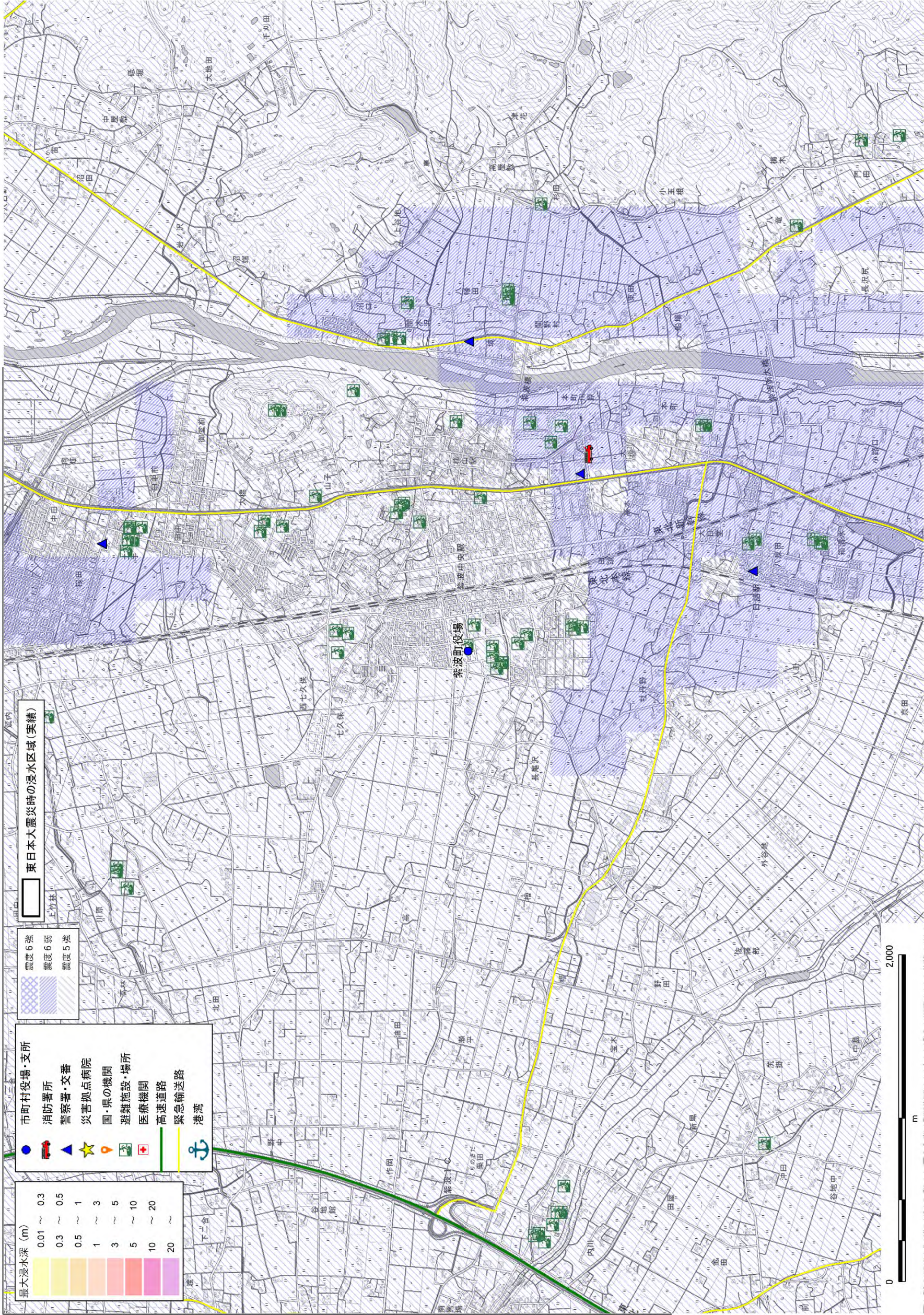
図 3.4.1-37 震度分布と防災上の重要施設の重ね合わせ図（紫波町）
