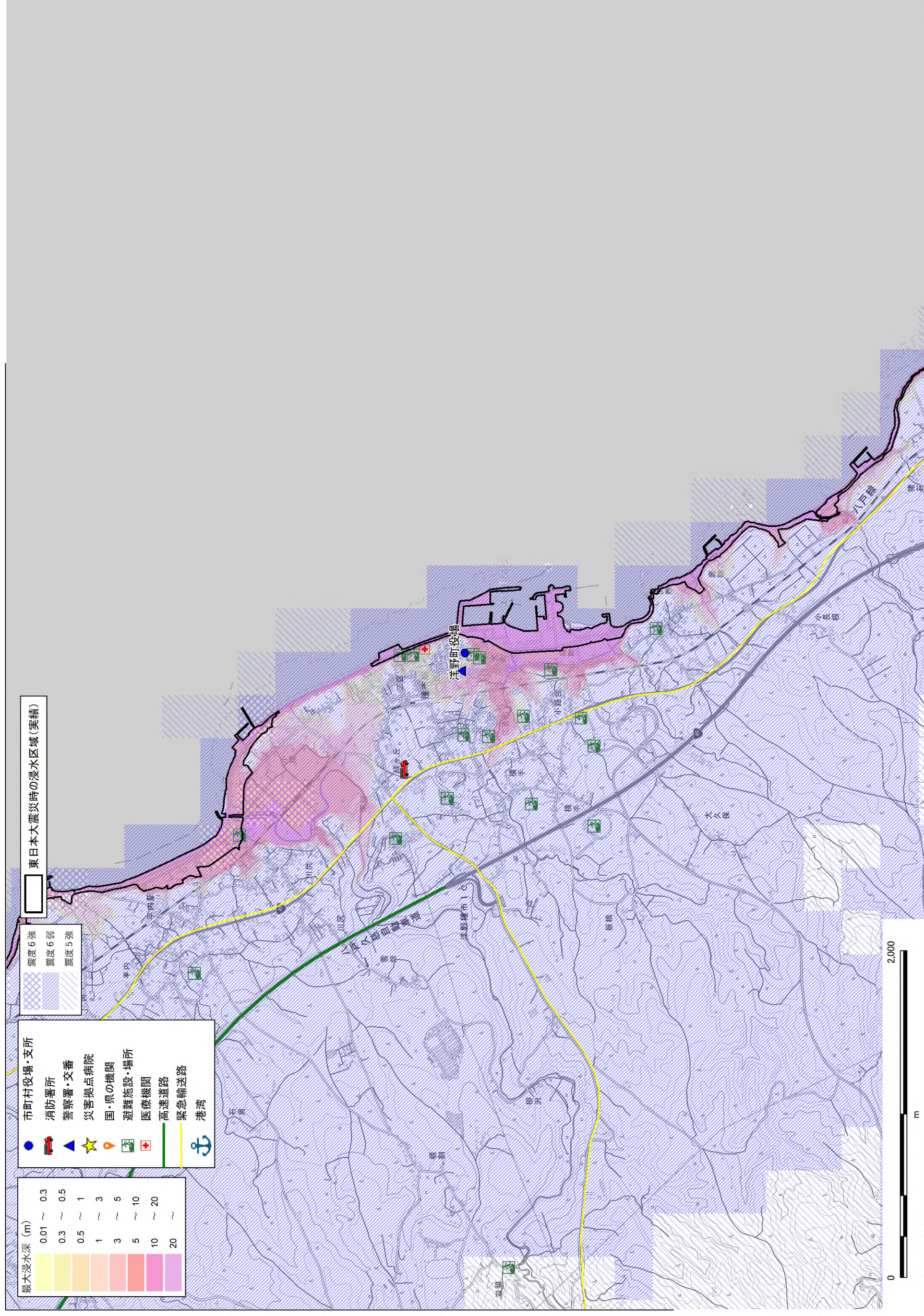
図 3.4.1-1 浸水深・震度分布と防災上の重要施設の重ね合わせ図 (洋野町)
