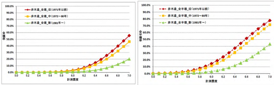
全壊率曲線
