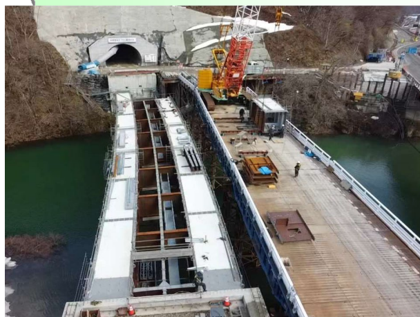
西和賀町：一般国道107号大石地区 トンネルによる災害復旧事業 (令和7年3月時点)
