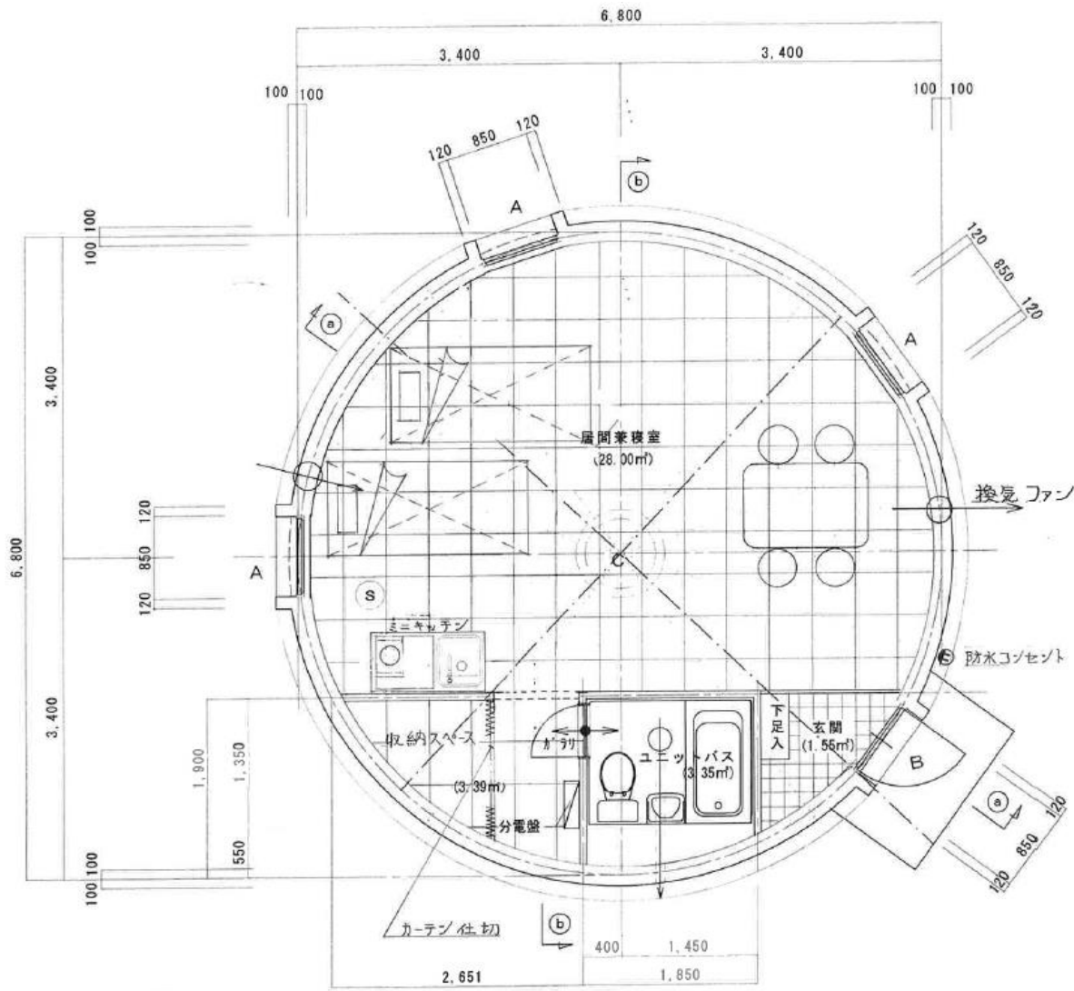
平面図 S=1:50
