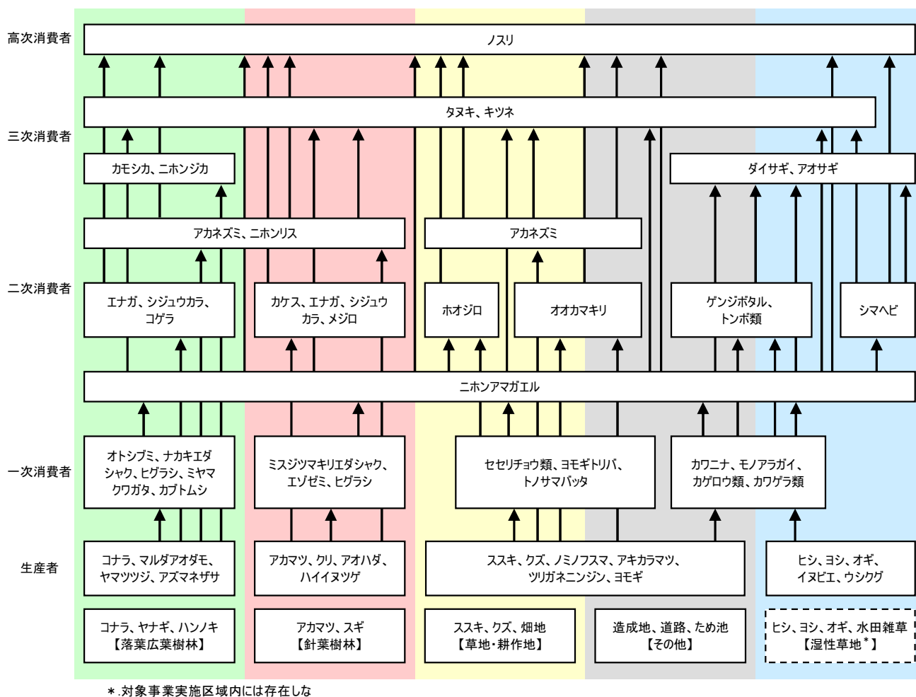
図 7.9-1 対象事業実施区域及びその周辺の生態系模式図
