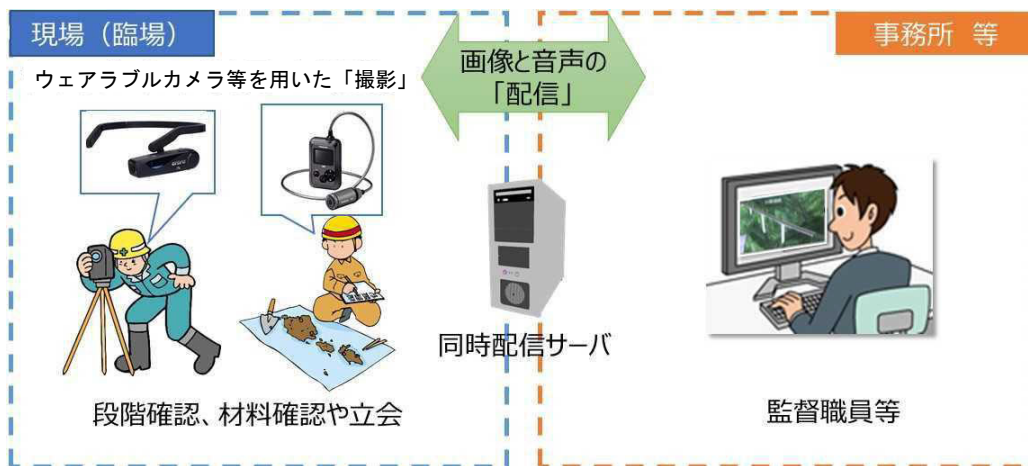
図 2-1 機器構成（例）
