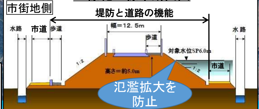
二線堤 標準断面図
