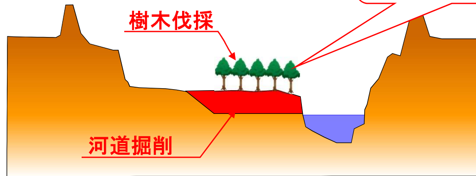
横断図(河道掘削イメージ) A-A断面
