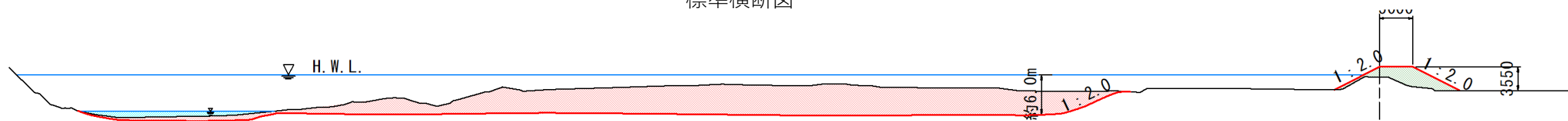
標準横断面図
