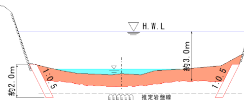
標準横断面図
