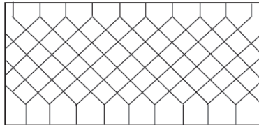
図3-2-4 谷 積
