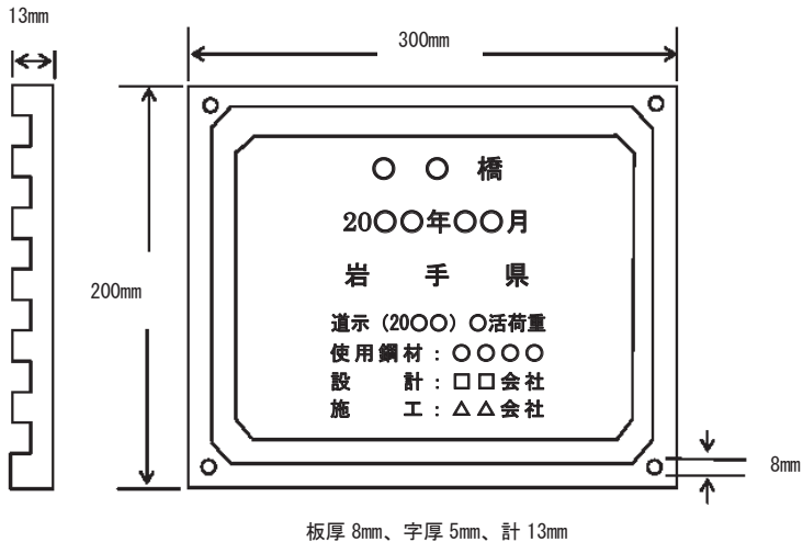
板厚 8mm、字厚 5mm、計 13mm 図3-2-2 銘板の寸法及び記載事項
