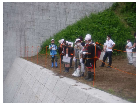
↑上乙茂の沢（4）砂防堰堤を見学！！
