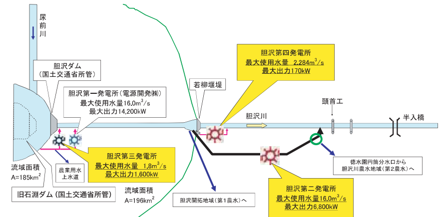
胆沢川を利用する発電所の取水模式図
