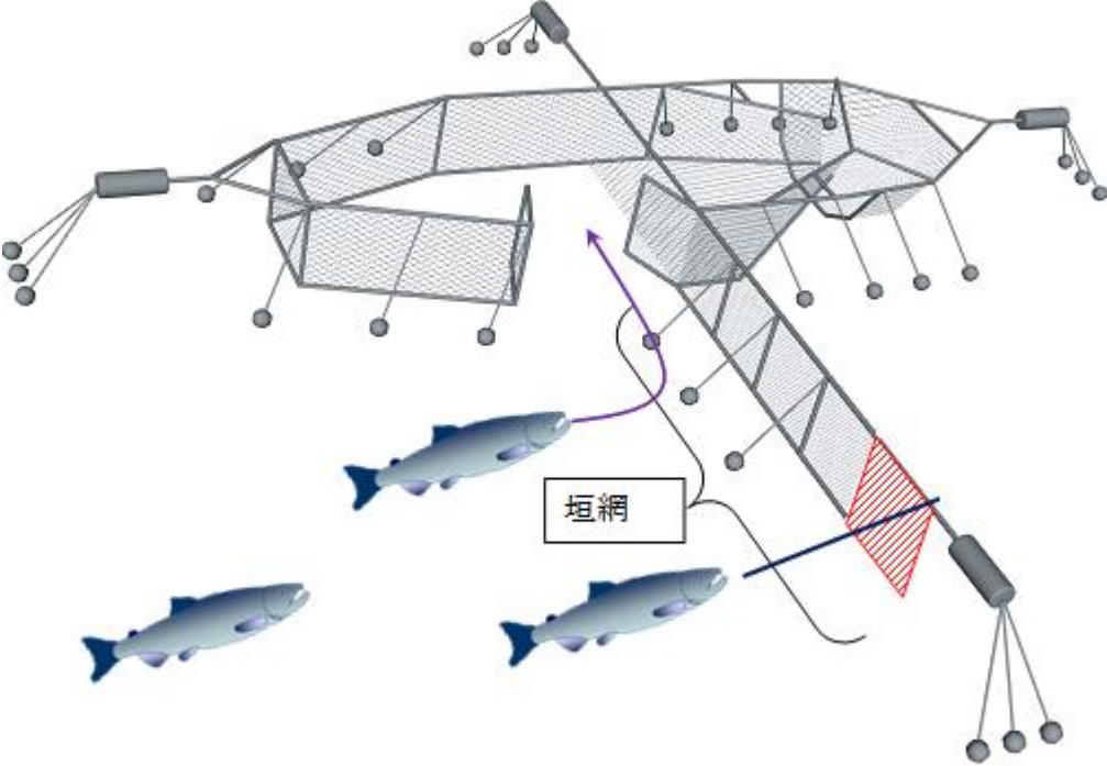
定置網の模式図
