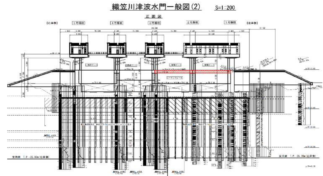
正面図
