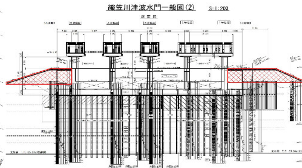
正面図
