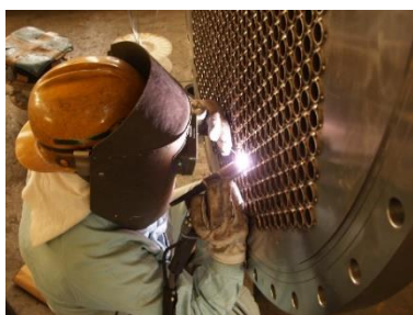
溶接作業
