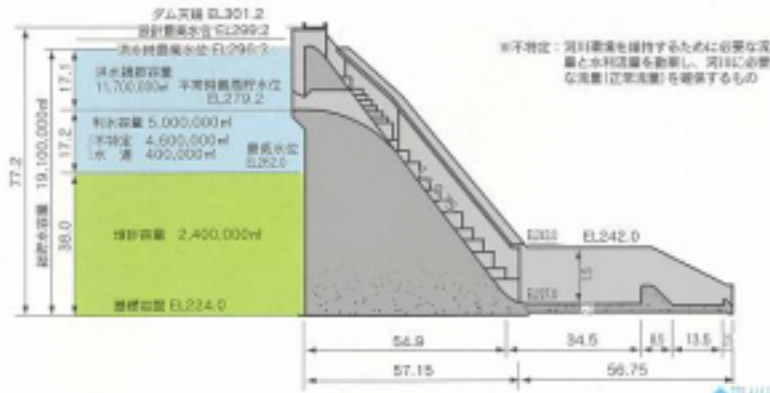
ダムの標準断面図および容量配分図 (単位: m)
