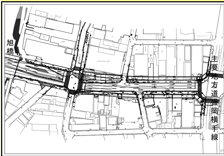
起点側
