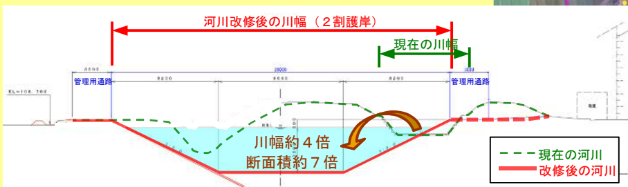
【砂子田橋上流付近の横断面図】
