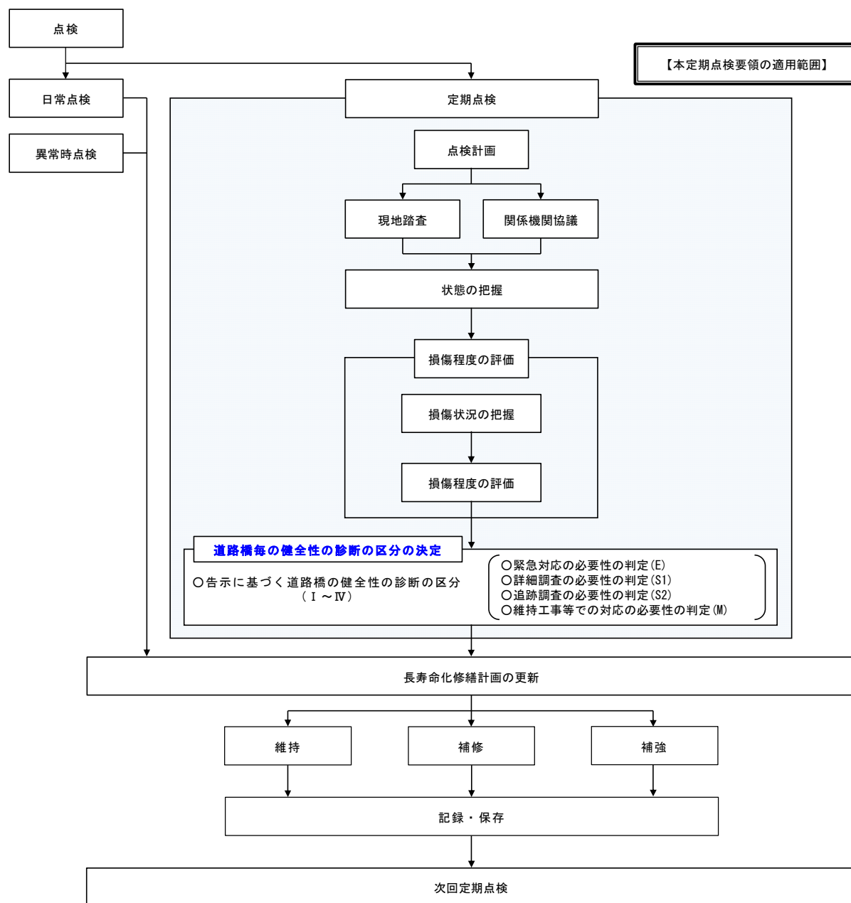
図－2. 3. 1 橋梁点検の流れ
