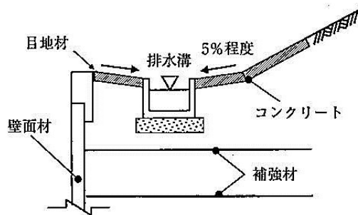
補強土壁頂部の排水溝の例
