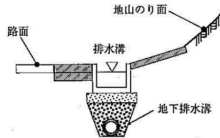
路面の側溝の例
