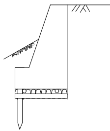
胴木基礎
