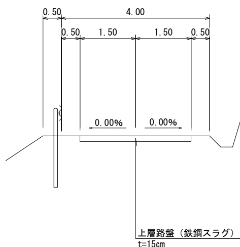
鉄鋼スラグ路盤工 標準断面図（岩部）
