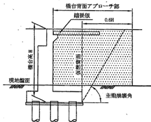
(a) 一般の橋台の場合
