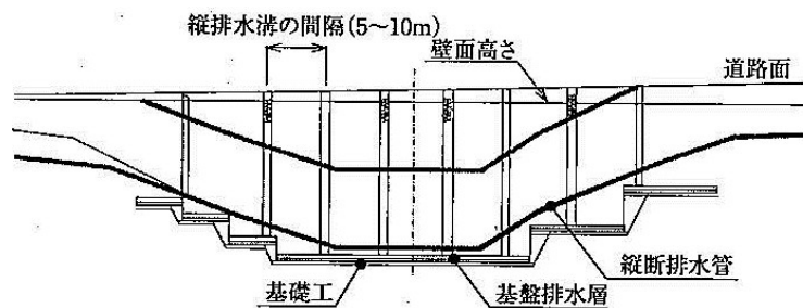
地下排水工の例（擁壁正面図）
