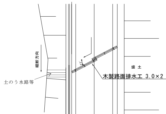
幅員4mで直線の盛土箇所の施工例
