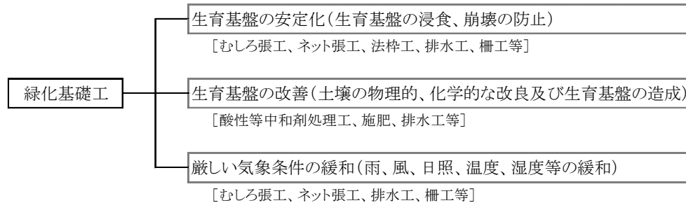
図4-4 緑化基礎工の目的による分類
