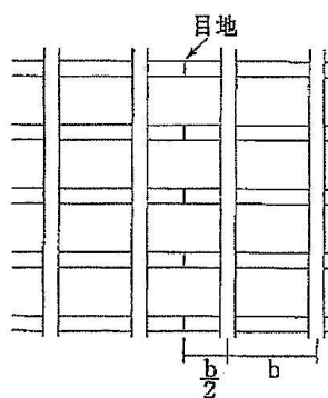
a) 横梁の中間への設置する場合
