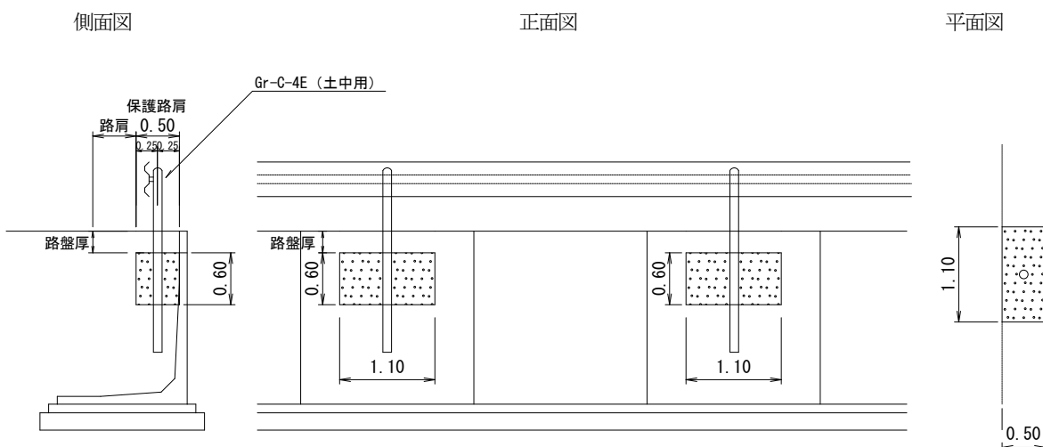
L型プレキャスト擁壁ガードレール基礎コンクリート施工図
