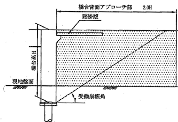
(b) 背面受働抵抗を考慮する橋台の場合
