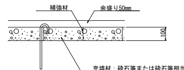
図一 路盤補強工構造図（参考図）
