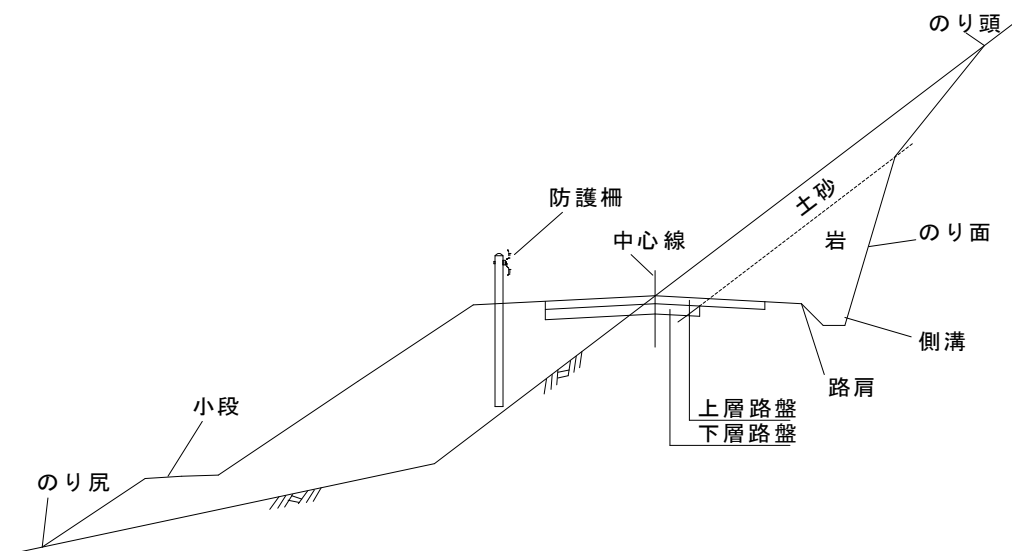
図 土工構造物の構造
