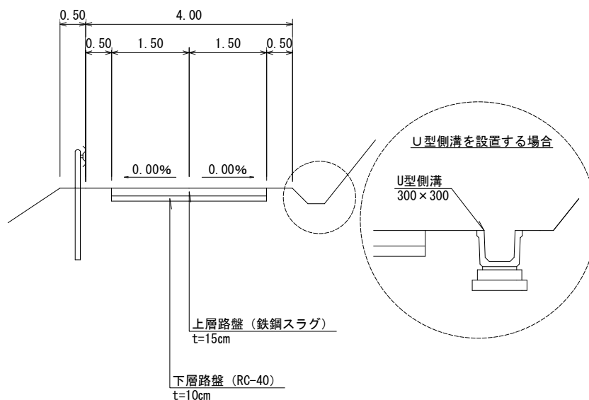
鉄鋼スラグ路盤工 標準断面図（土砂部）
