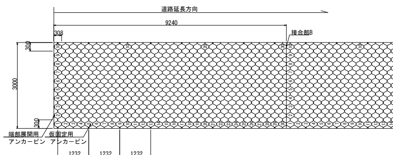
相互接合部詳細
