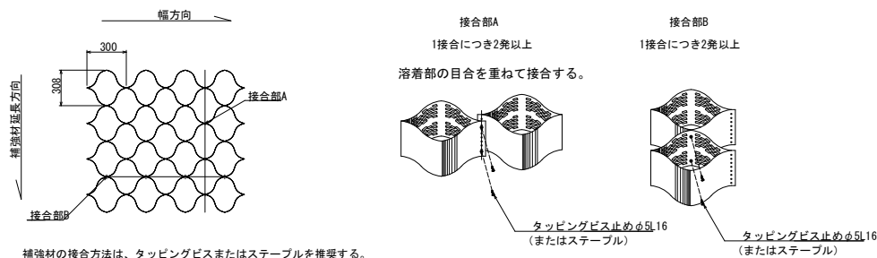
詳細断面
