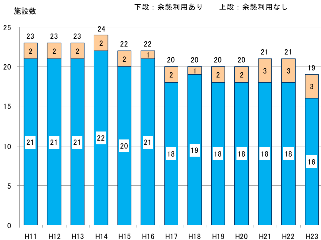
図-10 ごみ焼却施設の余熱利用の推移
