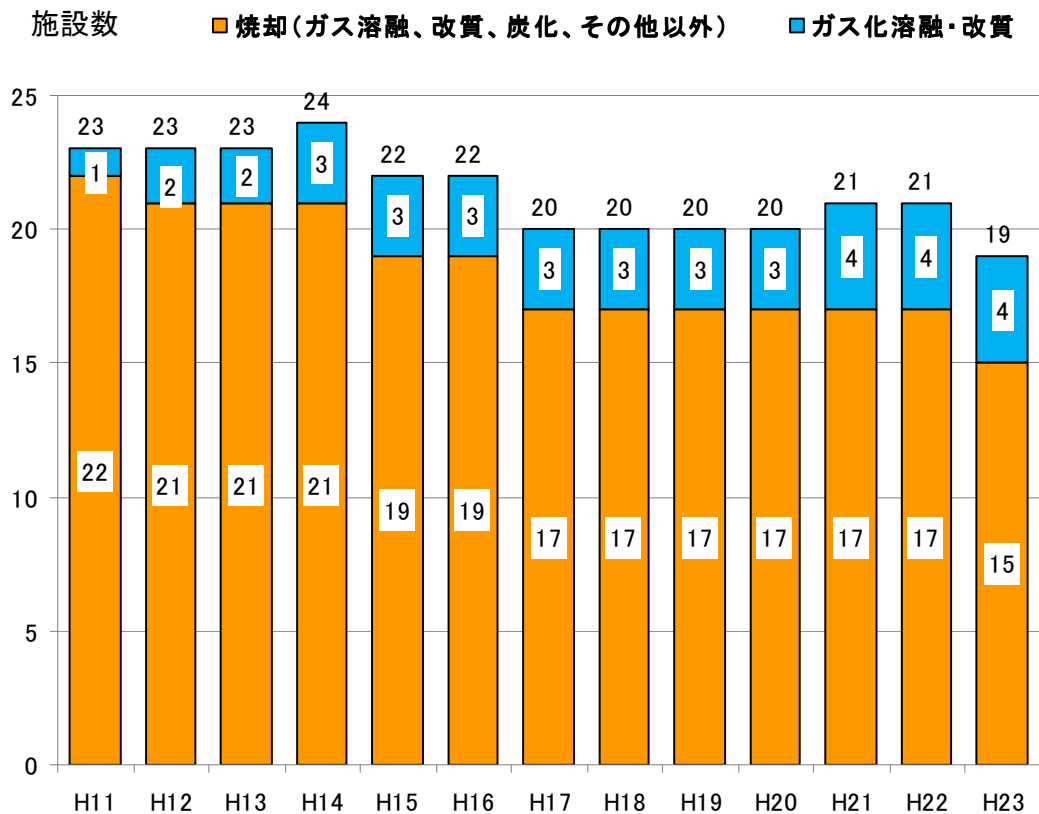
図－7 ごみ焼却施設の種類の施設数の推移
