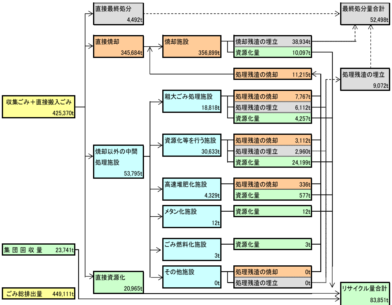
図-5 ごみの処理のフロー (単位: トン)
