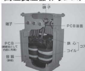
高圧変圧器(トランス)
